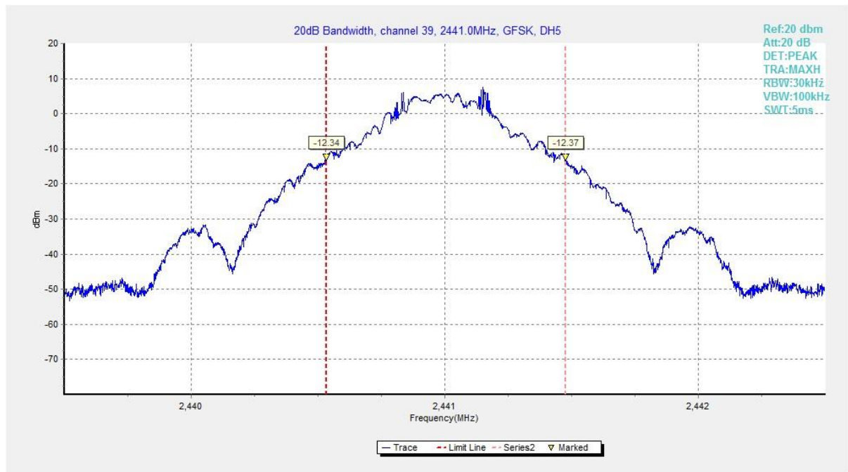
Fig. 62 20dB Bandwidth (GFSK, Ch 39)
