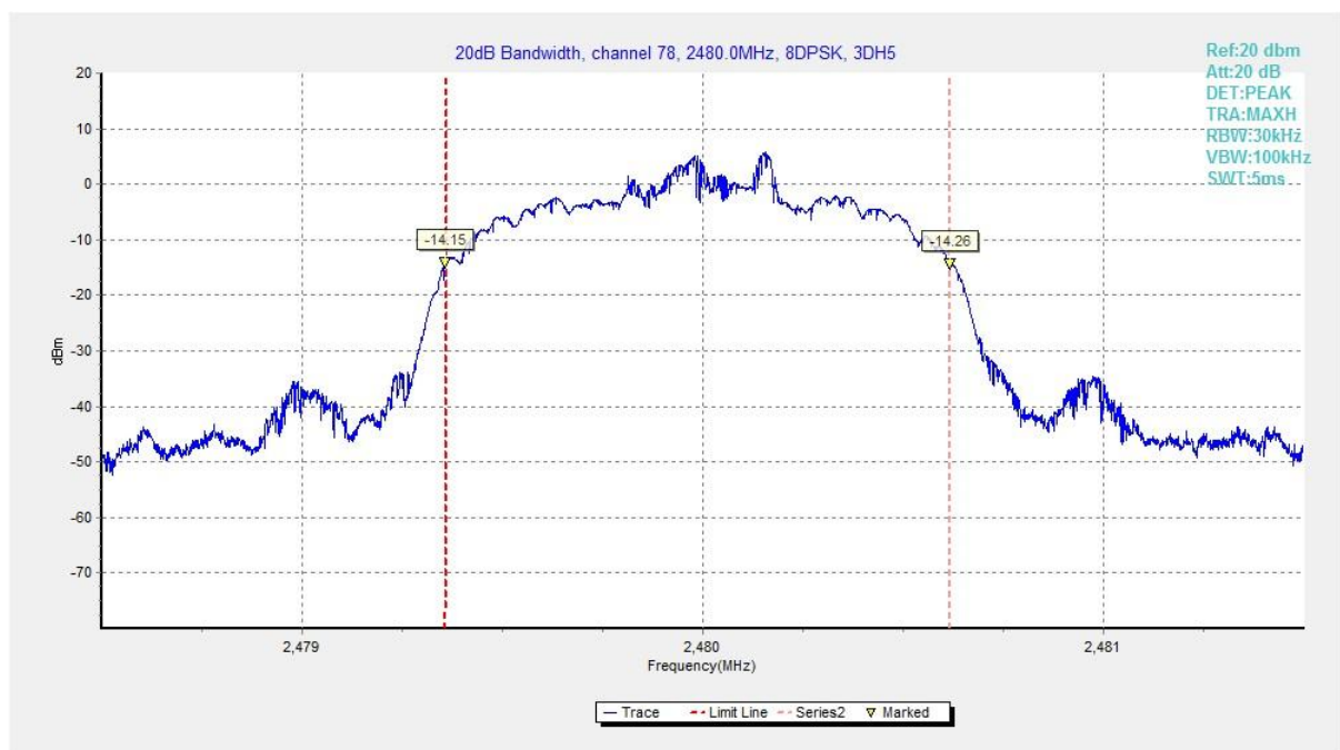
Fig. 69 20dB Bandwidth (8DPSK, Ch 78)
