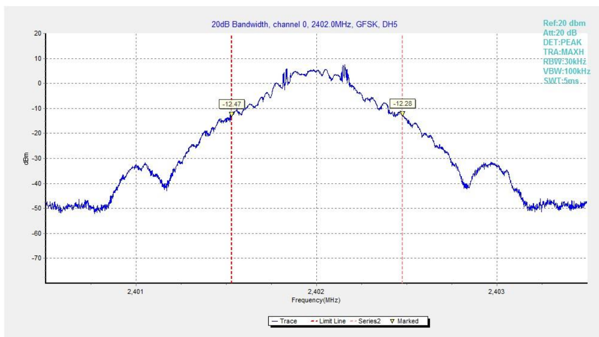
Fig. 61 20dB Bandwidth (GFSK, Ch 0)
