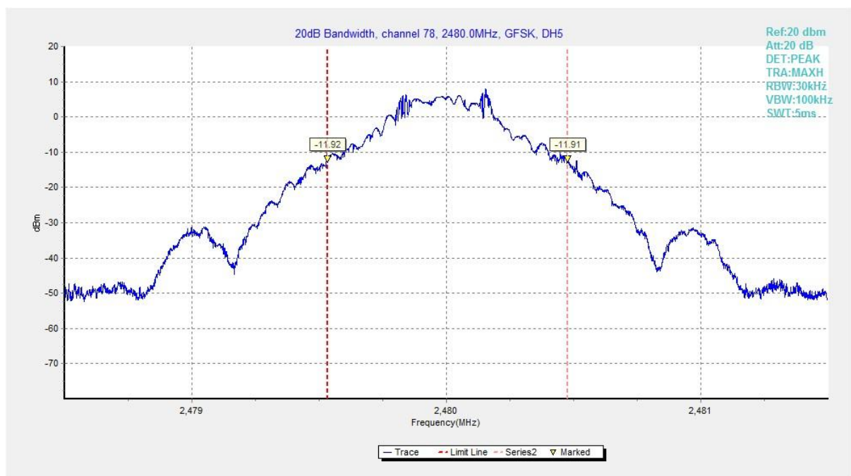
Fig. 63 20dB Bandwidth (GFSK, Ch 78)
