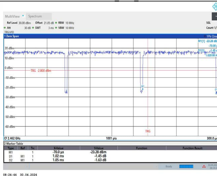
11AX20MIMO_Ant2_2462
