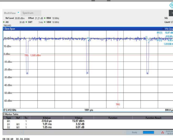
11AX20MIMO_Ant1_2412
