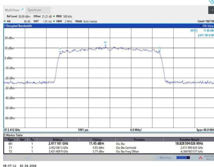
11AX20MIMO_Ant1_2412
