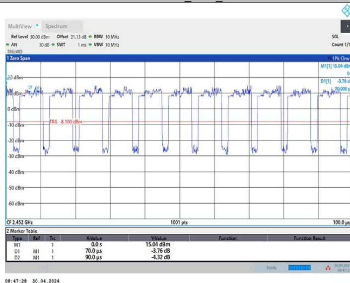
11AX40MIMO_Ant1_2452
