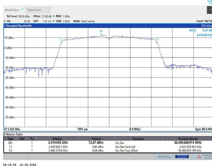
11N40MIMO_Ant2_2422
