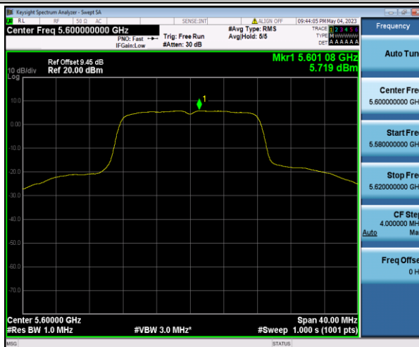
11A_Ant1_5600
