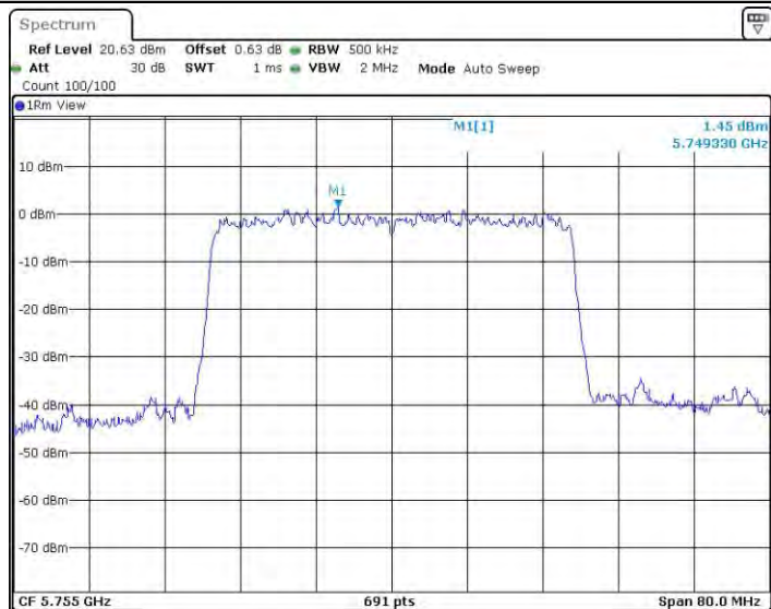
11AX40MIMO_Ant0_5755
