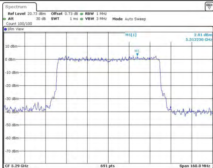
11AX80MIMO_Ant0_5290
