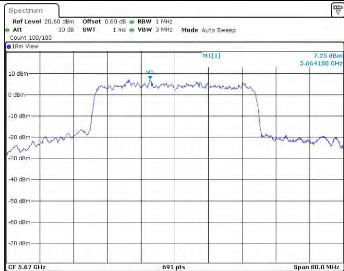
11AX40MIMO_Ant0_5670
