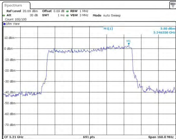
11AX80MIMO_Ant0_5210
