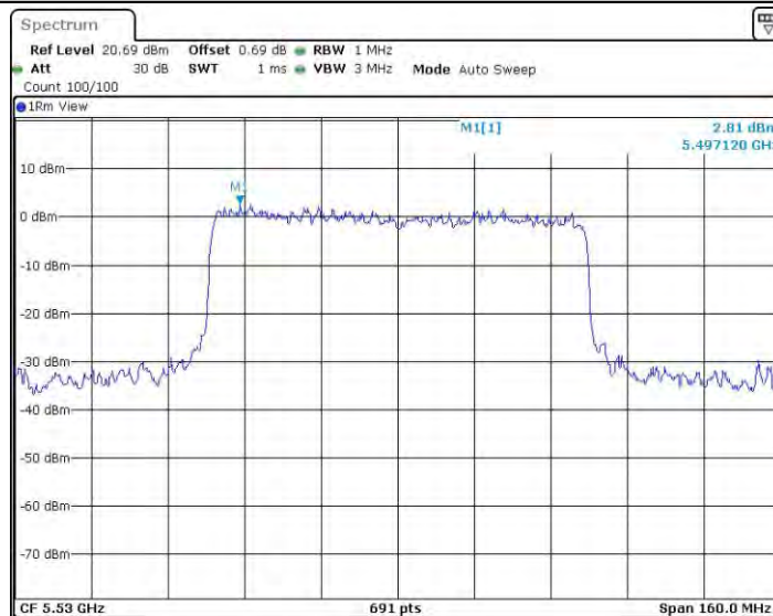
11AX80MIMO_Ant1_5530
