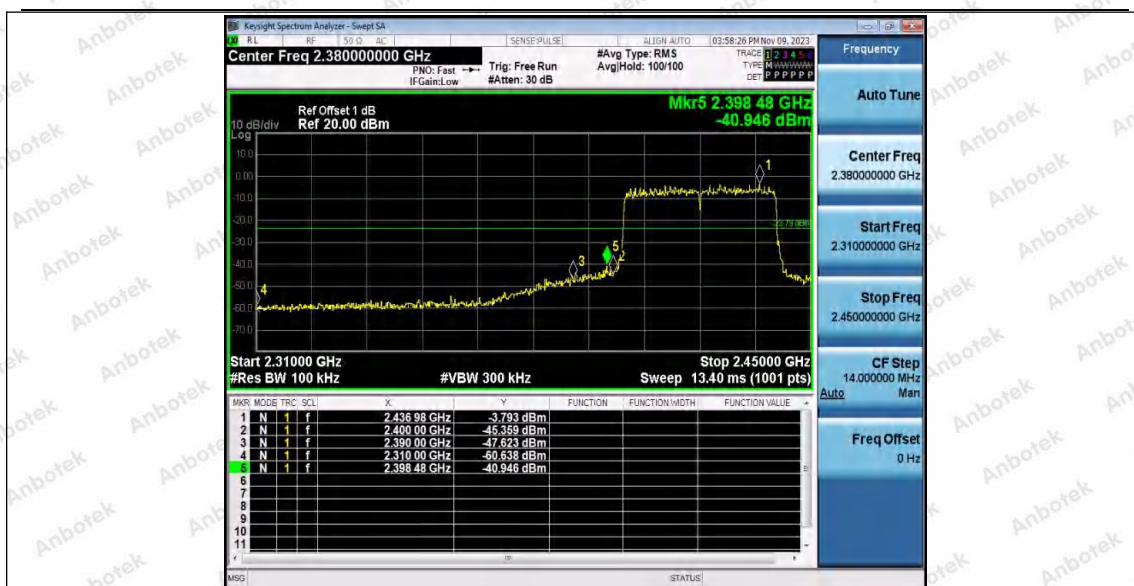
11AX40SISO_Ant2_Low_2422
