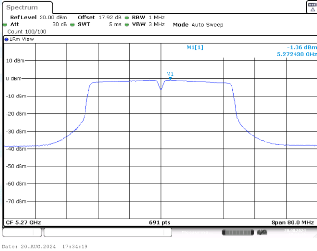
11N40SISO-Ant3-5270-PASS
