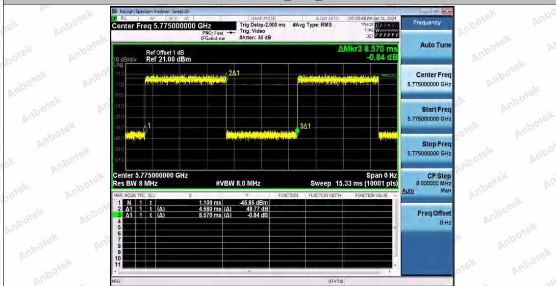
11AX80ISO_Ant1_5775
