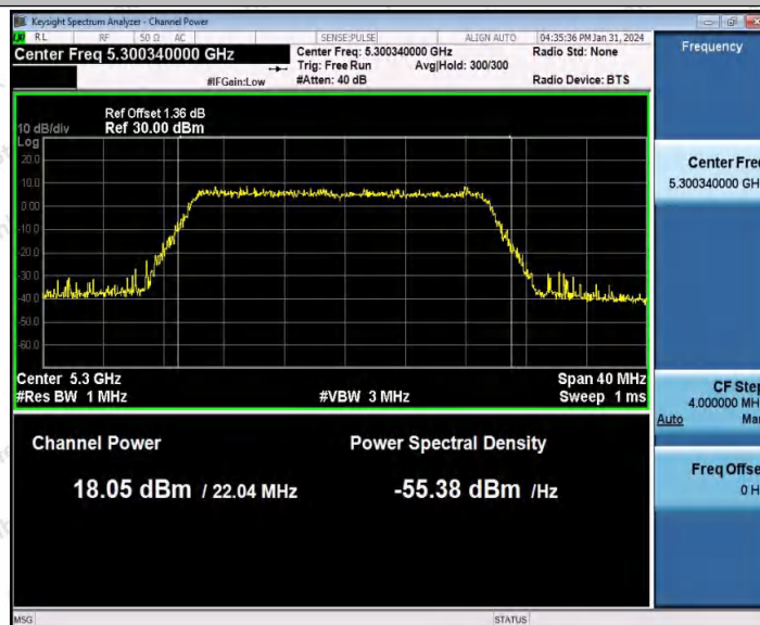
11AX20SISO_Ant1_5300
