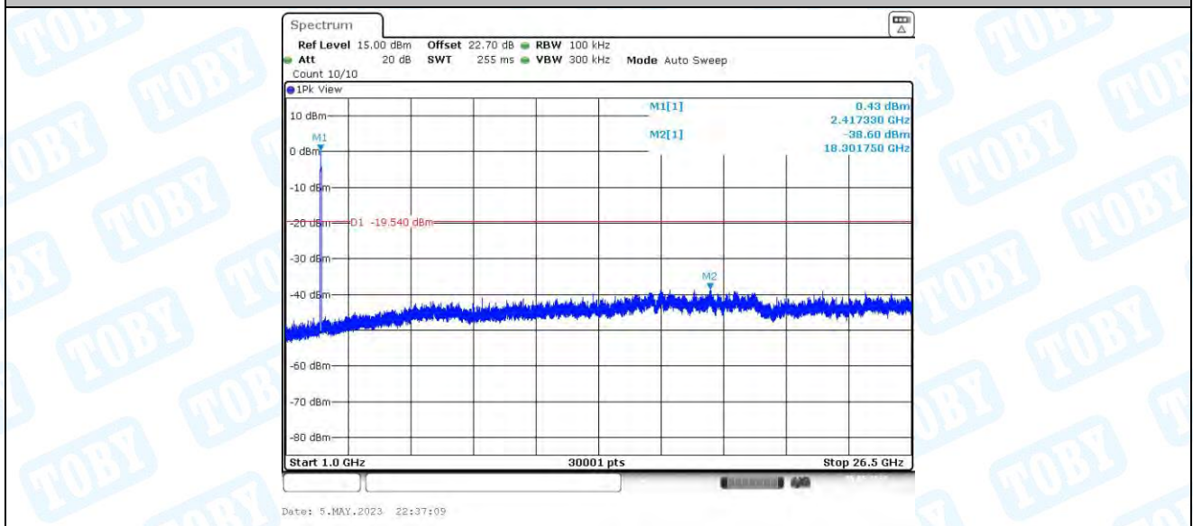
11N40MIMO_Ant4_2422_0~Reference
