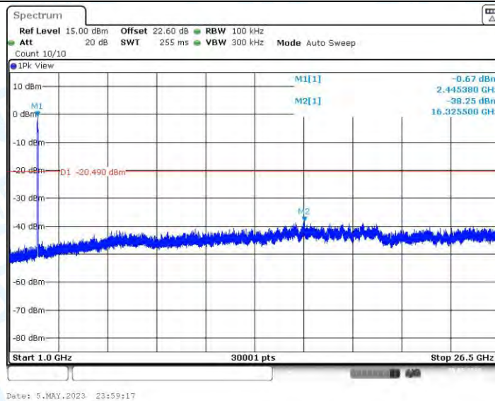
11AX40MIMO_Ant4_2452_0~Reference
