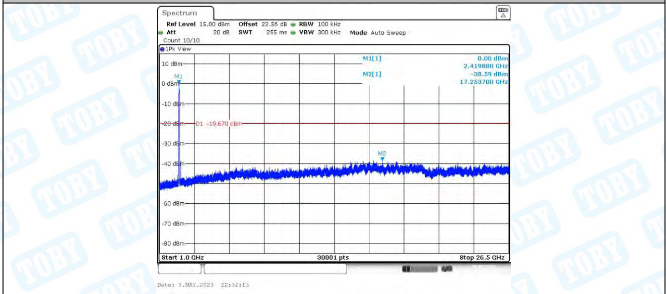
11N40MIMO_Ant2_2422_0~Reference
