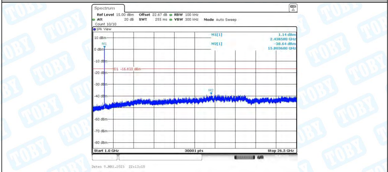
11N20MIMO_Ant3_2437_0~Reference
