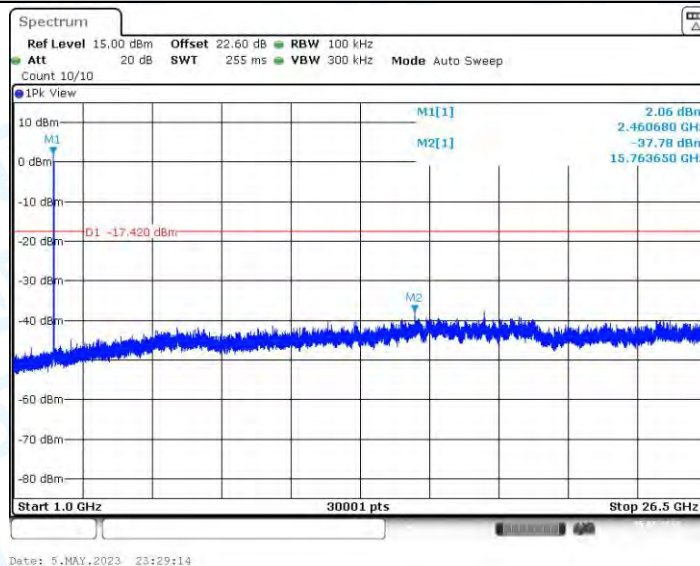
11AX20MIMO_Ant4_2462_0~Reference
