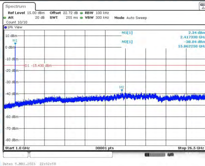
11N20MIMO_Ant3_2412_0~Reference
