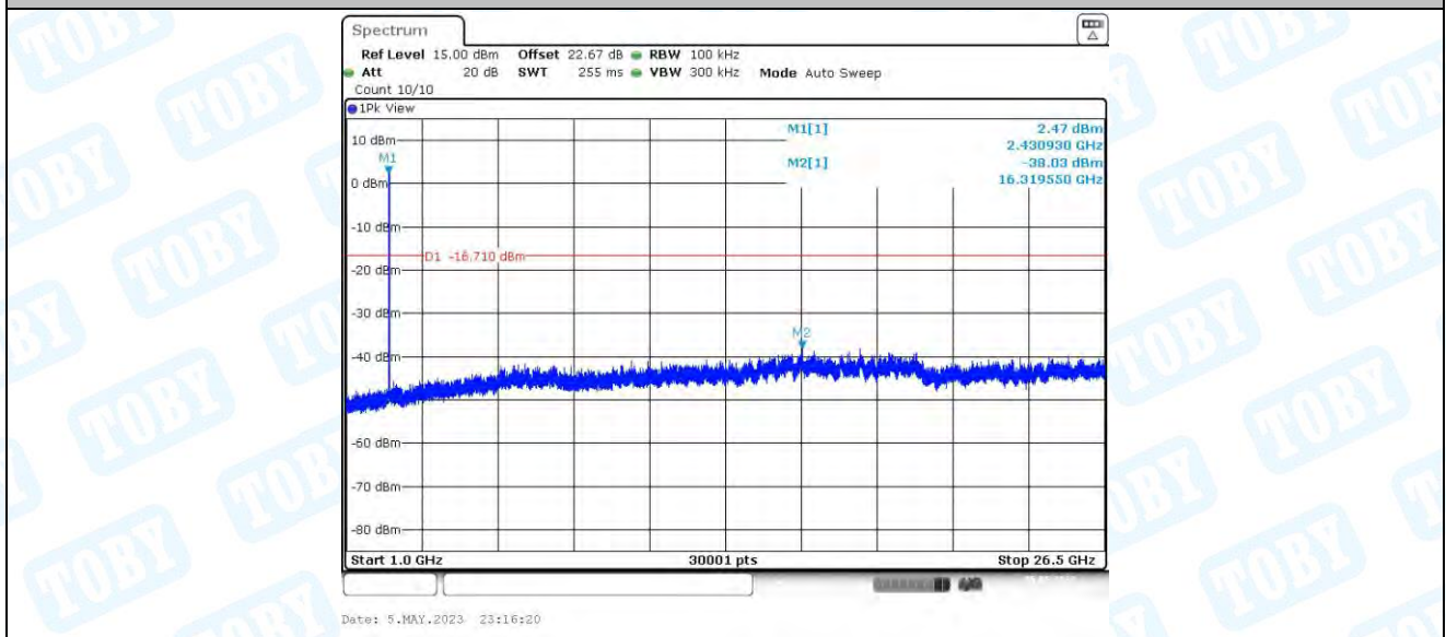
11AX20MIMO_Ant3_2437_0~Reference
