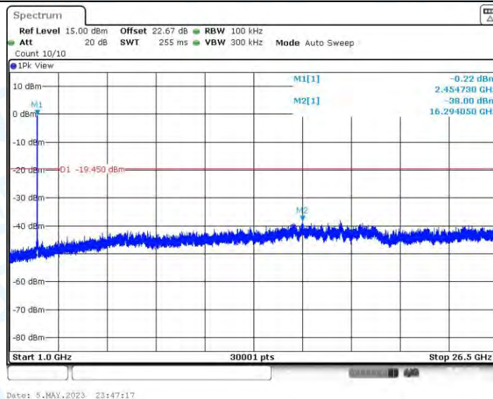
11AX40MIMO_Ant3_2437_0~Reference
