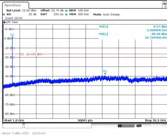
11AX20MIMO_Ant4_2412_0~Reference
