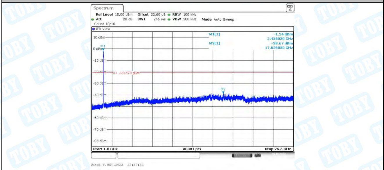
11N40MIMO_Ant4_2452_0~Reference
