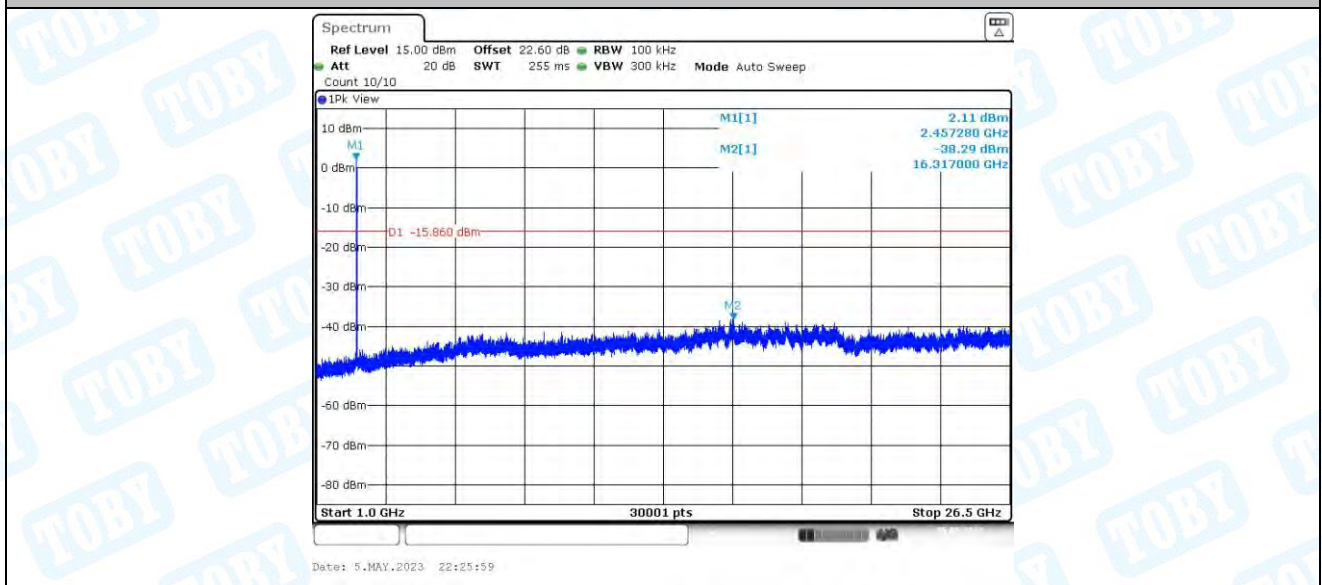
11N20MIMO_Ant4_2462_0~Reference
