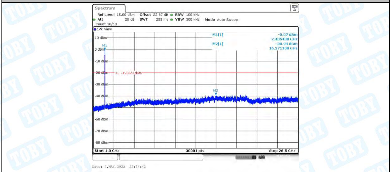
11N40MIMO_Ant3_2422_0~Reference
