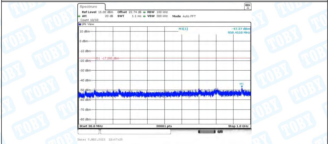
11N20MIMO_Ant4_2412_1000~26500
