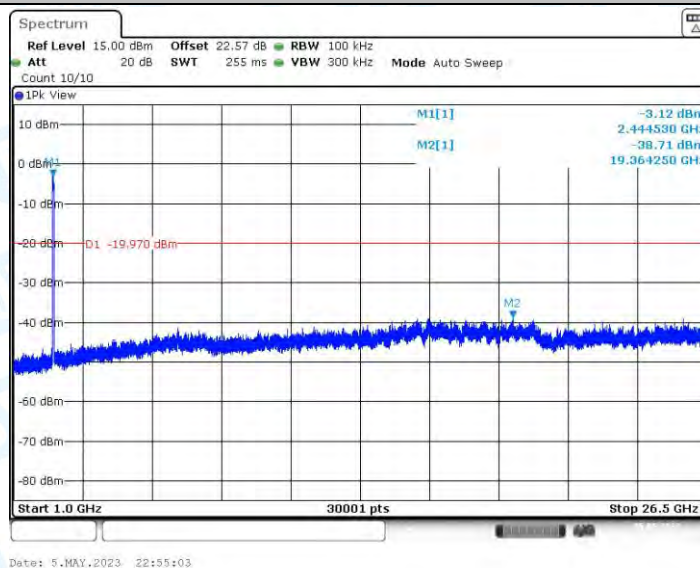
11N40MIMO_Ant3_2452_0~Reference
