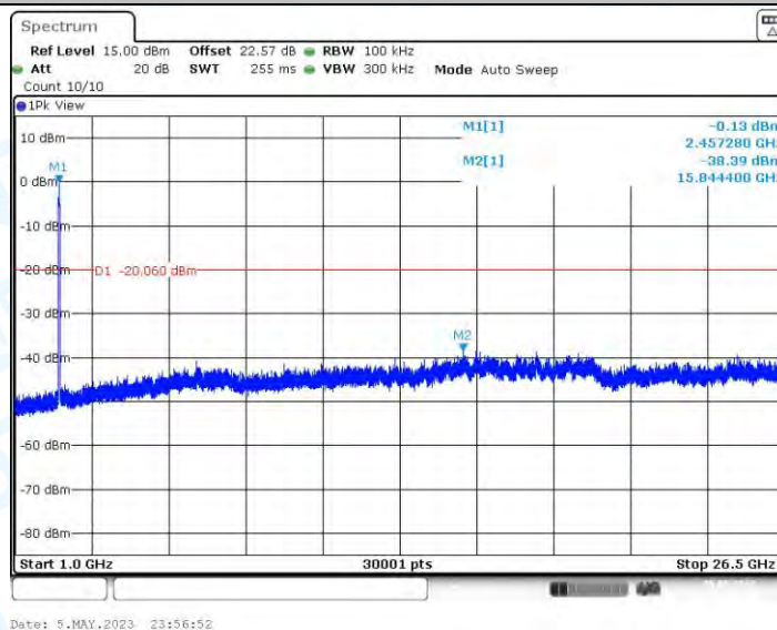
11AX40MIMO_Ant3_2452_0~Reference
