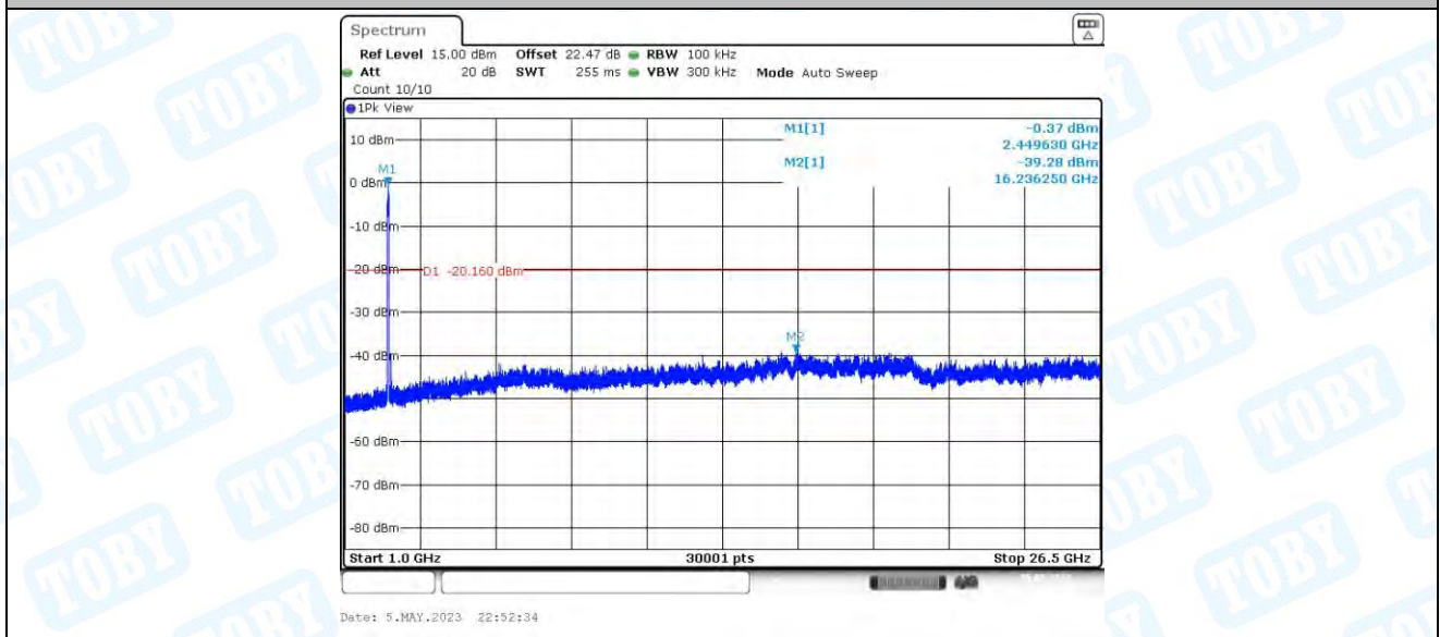
11N40MIMO_Ant2_2452_0~Reference
