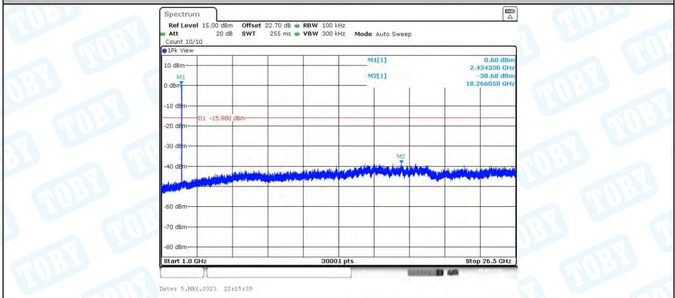
11N20MIMO_Ant4_2437_0~Reference
