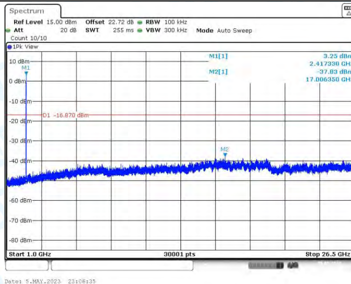
11AX20MIMO_Ant3_2412_0~Reference
