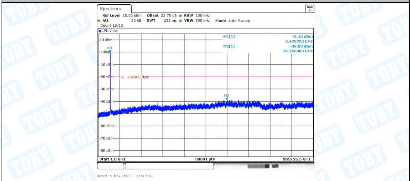
11AX40MIMO_Ant4_2437_0~Reference
