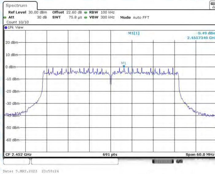
11AX40MIMO_Ant3_2452_30~1000
