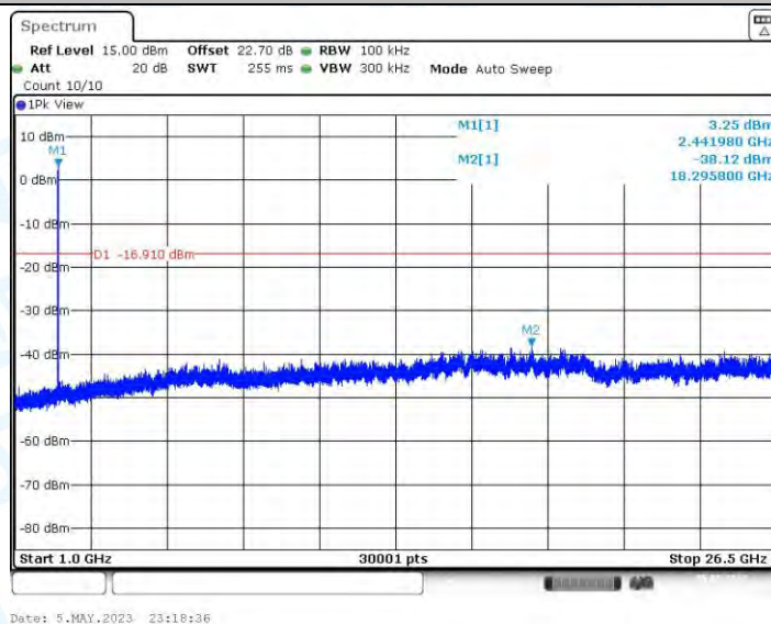
11AX20MIMO_Ant4_2437_0~Reference
