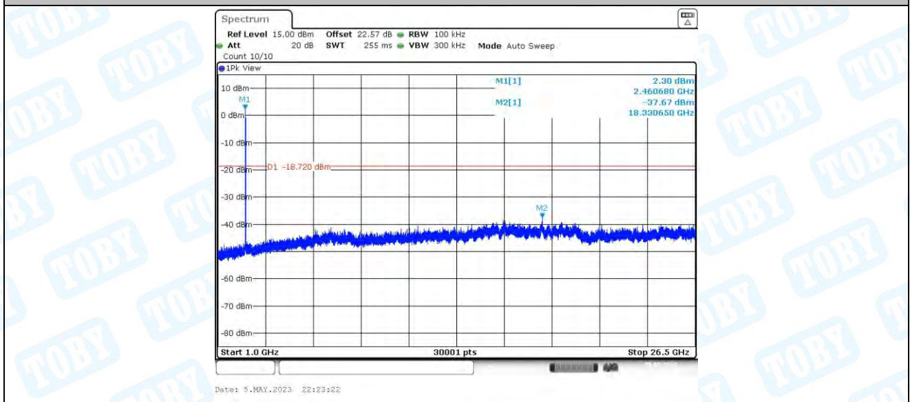
11N20MIMO_Ant3_2462_0~Reference
