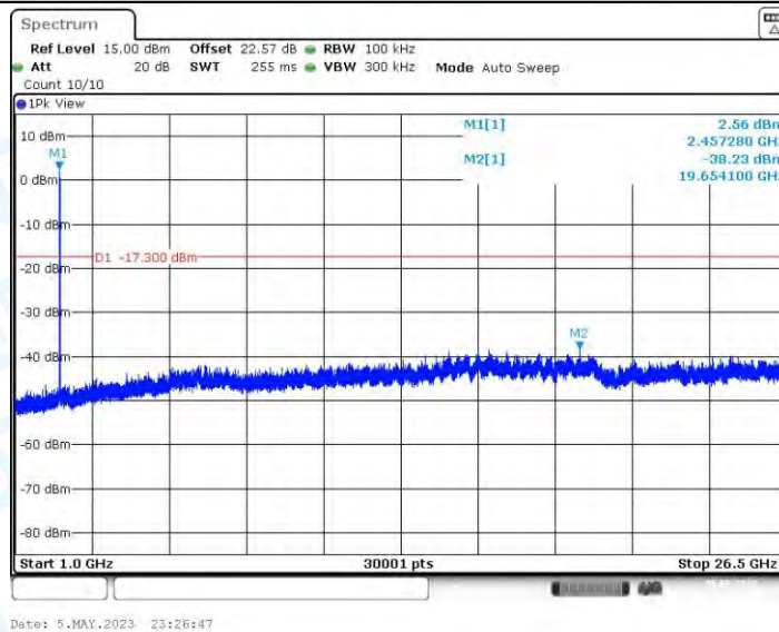
11AX20MIMO_Ant3_2462_0~Reference
