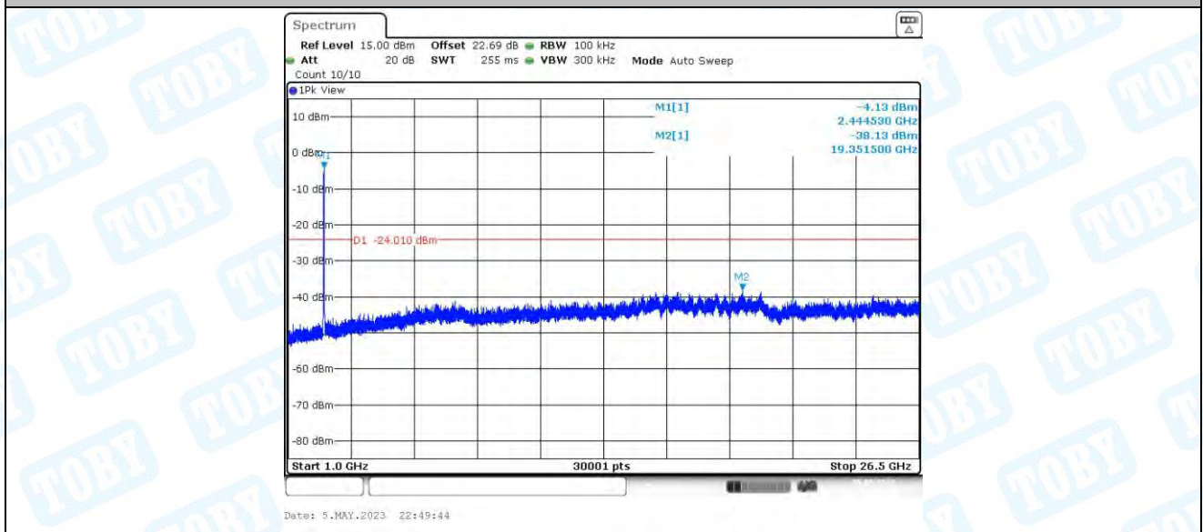
11N40MIMO_Ant1_2452_0~Reference
