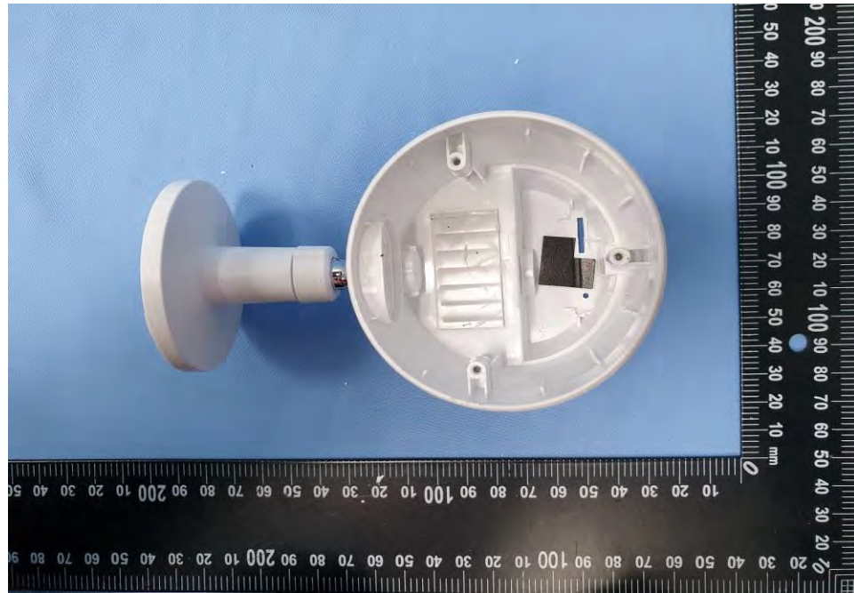
EUT Photo (31)
