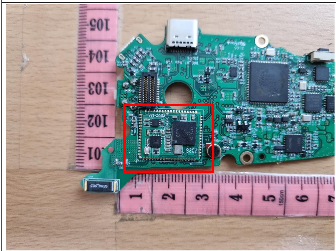
BT Module
