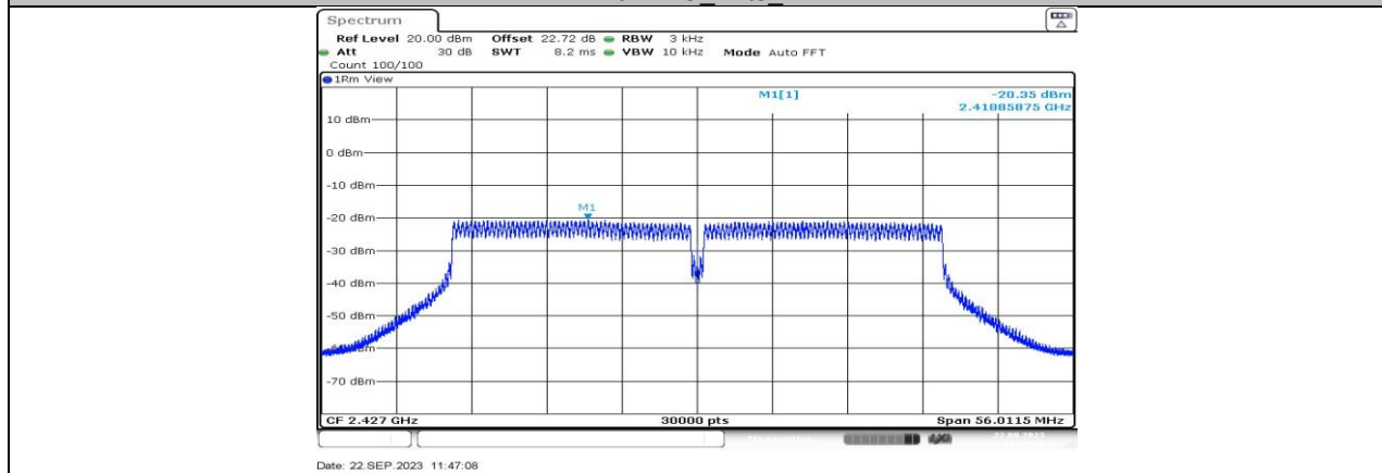
11N40MIMO_Ant4_2427
