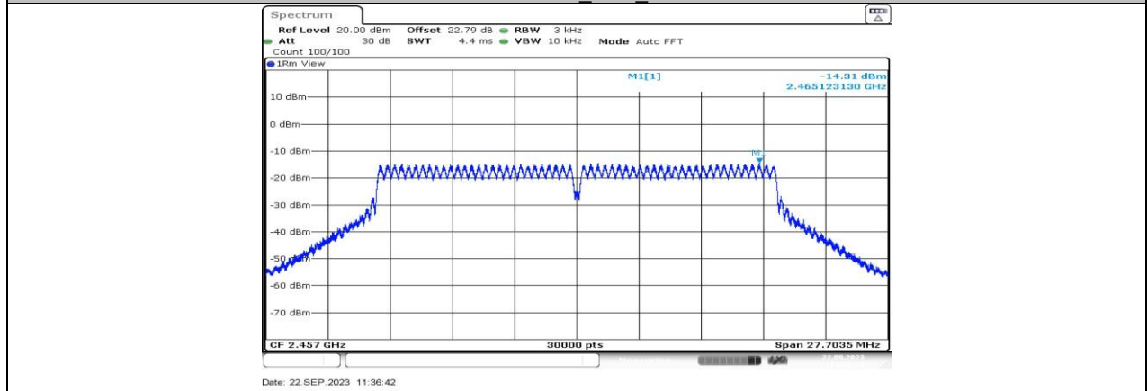
11N20MIMO_Ant3_2457
