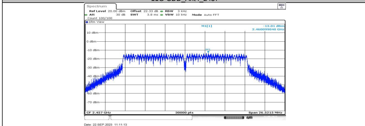
11G-CDD_Ant1_2457
