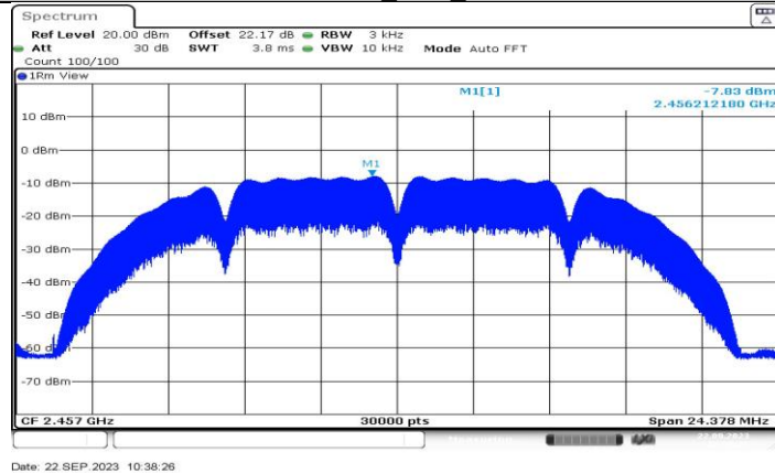
11B-CDD_Ant1_2457
