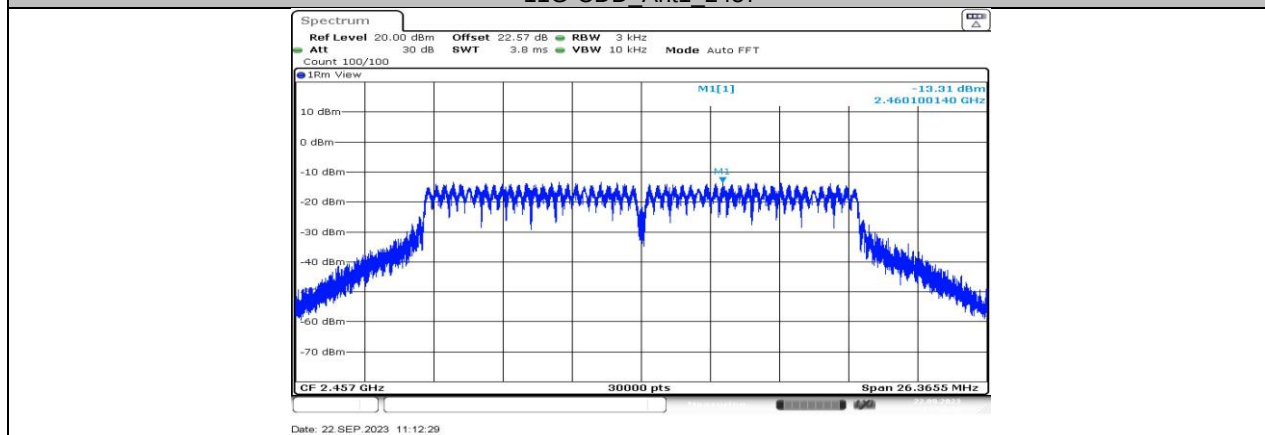
11G-CDD_Ant2_2457
