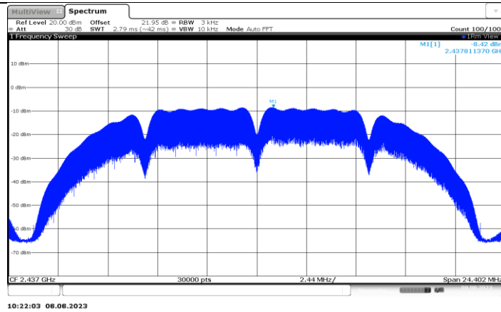
11B-CDD_Ant3_2437
