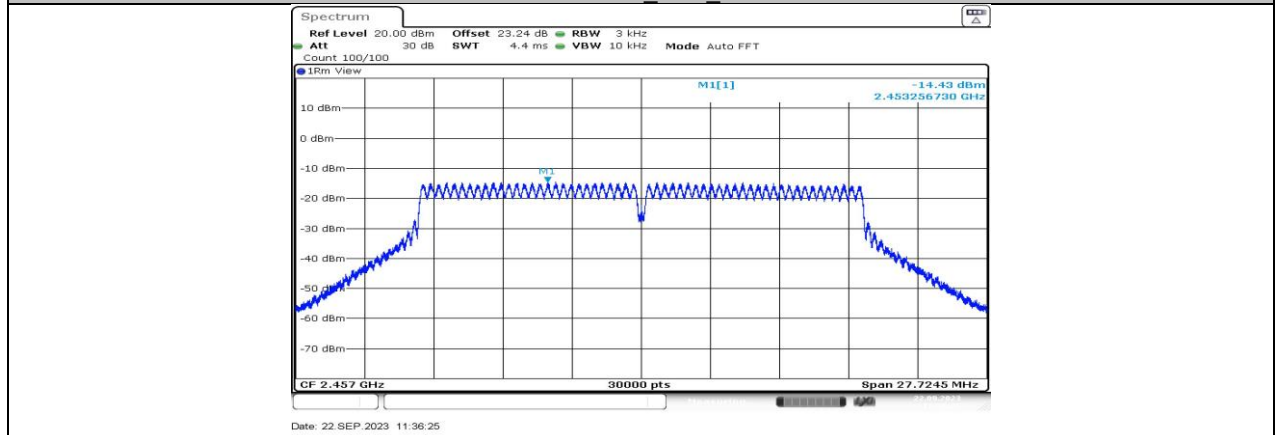
11N20MIMO_Ant2_2457
