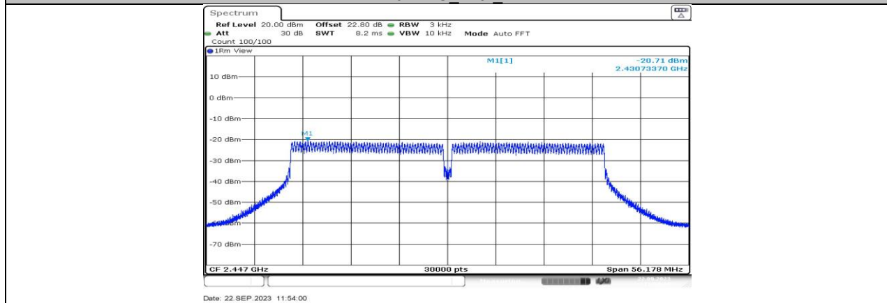
11N40MIMO_Ant3_2447
