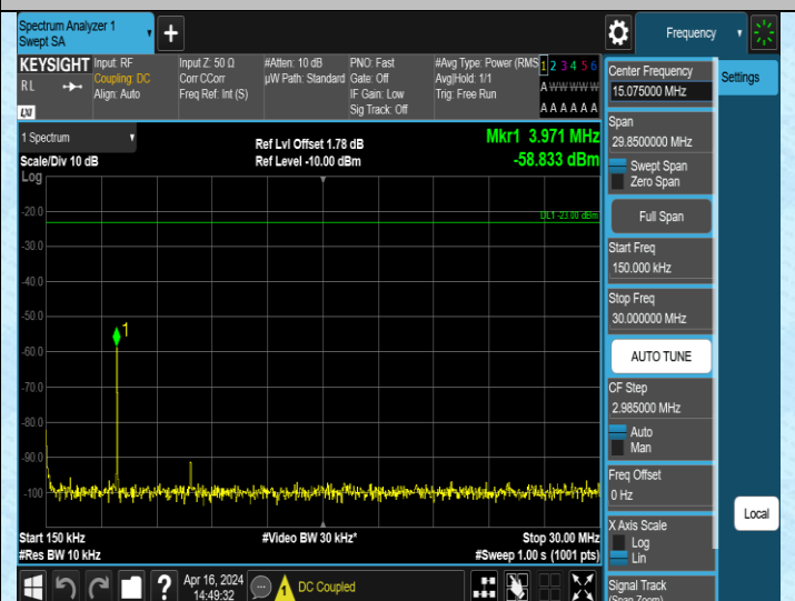
Band5 1.4MHz QPSK 20643 1RB#0 0.15~30 0.15~30
