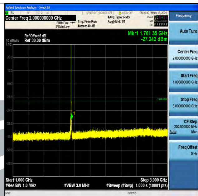
Band4 3MHz QPSK 20385 1RB#0 1000~3000 1000~3000
