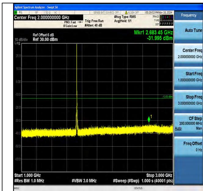
Band4 5MHz QPSK 20175 1RB#0 1000~3000 1000~3000
