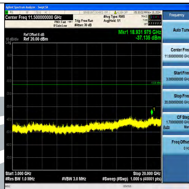
Band4 5MHz QPSK 20175 1RB#0 3000~20000 3000~20000
