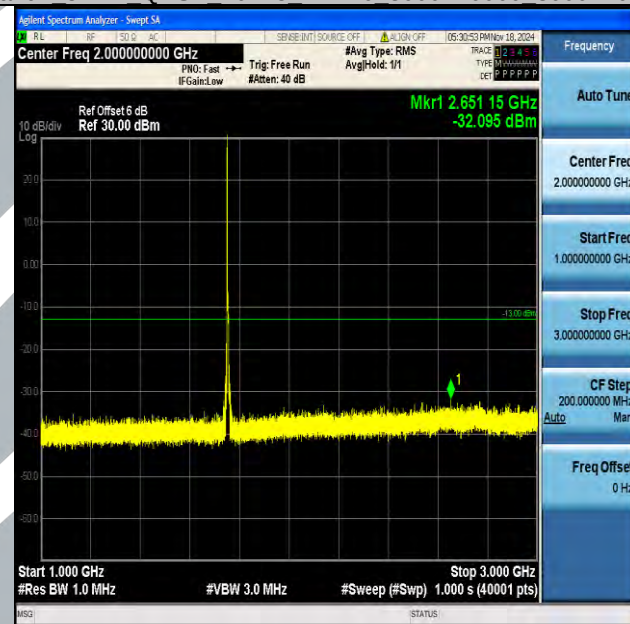
Band4 5MHz QPSK 20375 1RB#0 1000~3000 1000~3000
