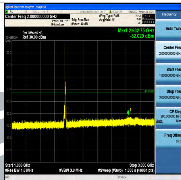
Band4 10MHz QPSK 20350 1RB#0 1000~3000 1000~3000
