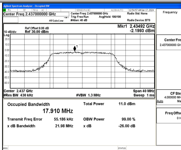
11N20MIMO-Ant1-2437
