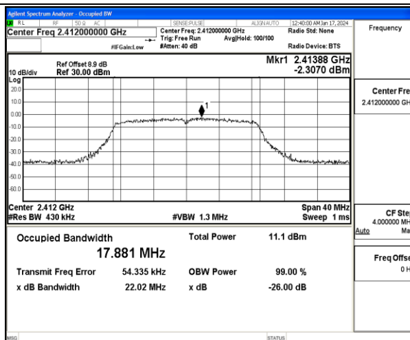
11N20MIMO-Ant1-2412
