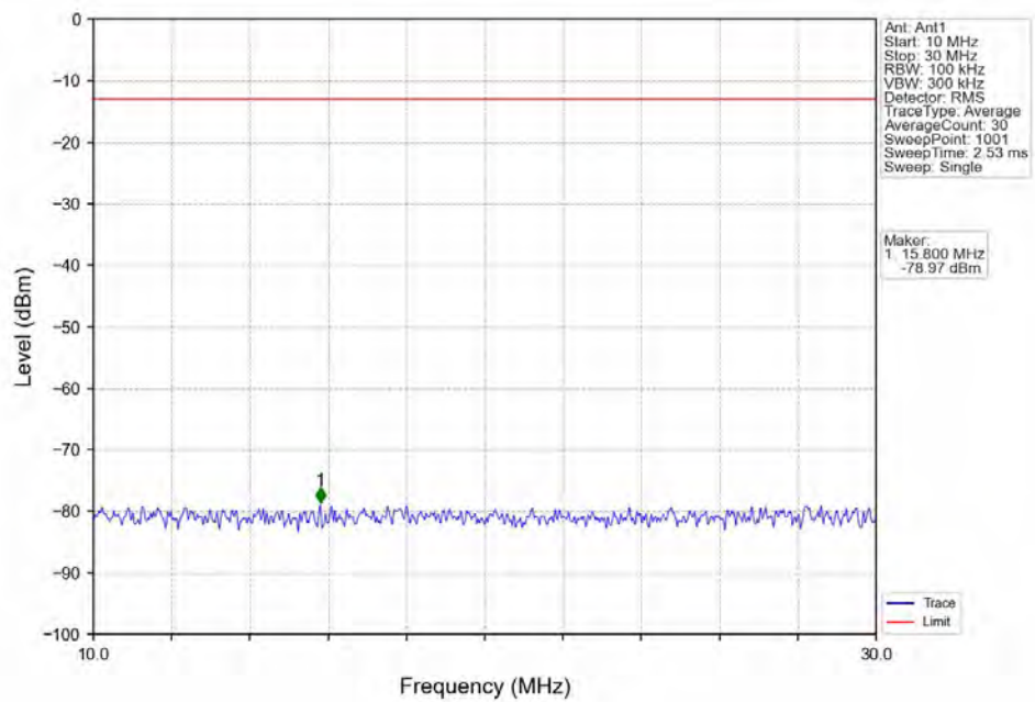
Band4_20MHz_QPSK_LCH_1720MHz_RB_1_0_NTNV
