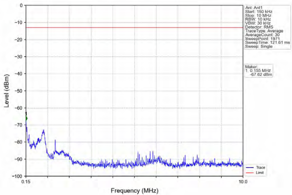
Band4_10MHz_QPSK_HCH_1750MHz_RB_1_0_NTNV
