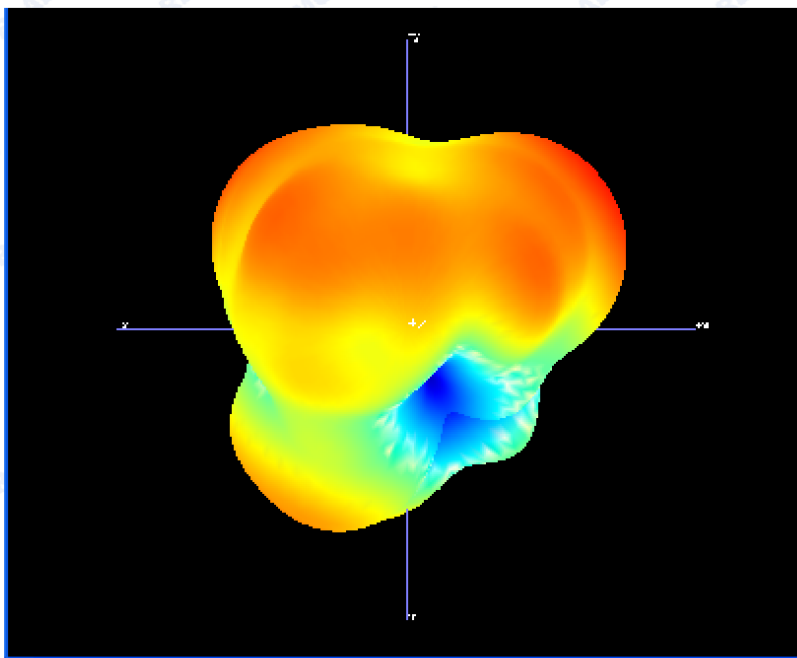
2450MHz
