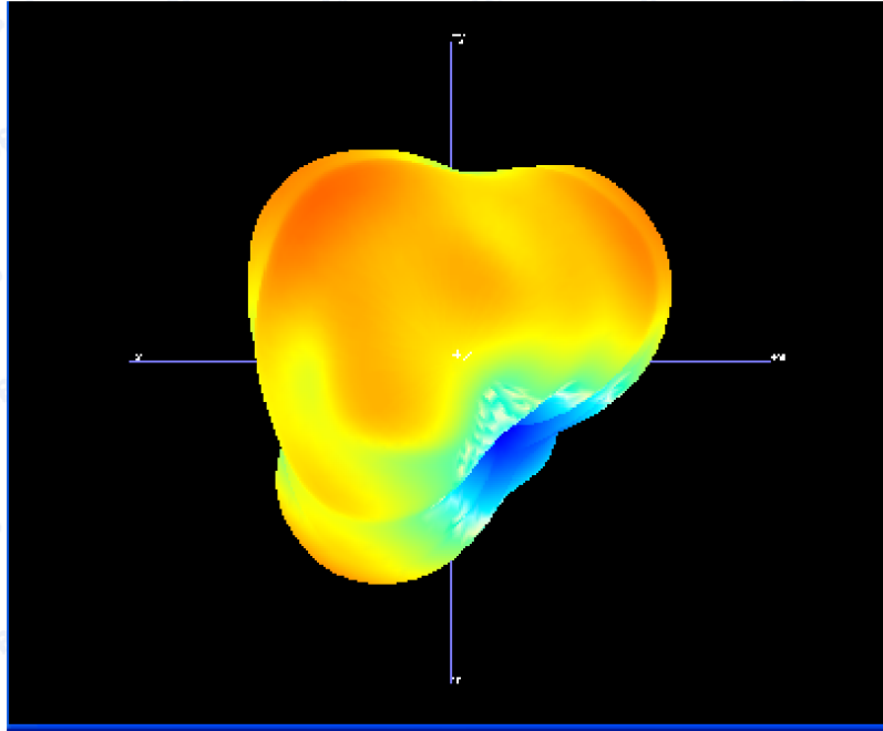
2400MHz
