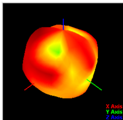
WIFI 5.8G天线3D图
