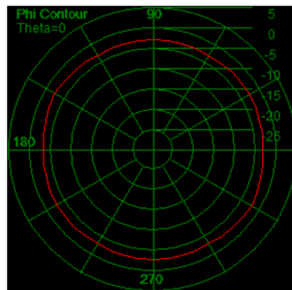
天线2D图H面
