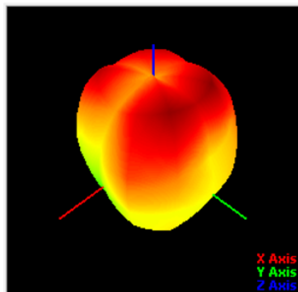
WIFI 5.8G天线3D图
