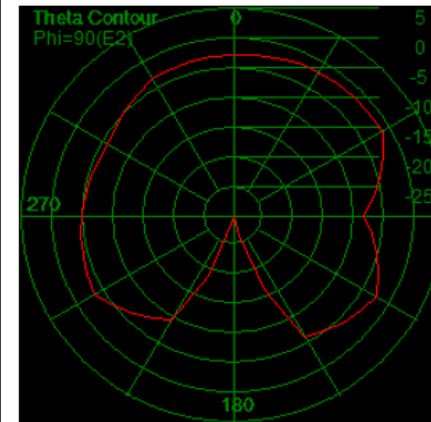
E2面
