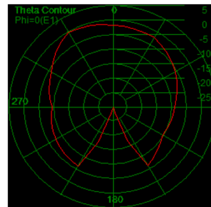
E1面
