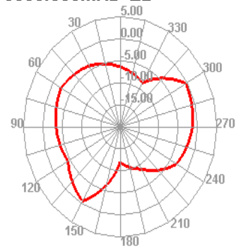
5550.000MHz E2
