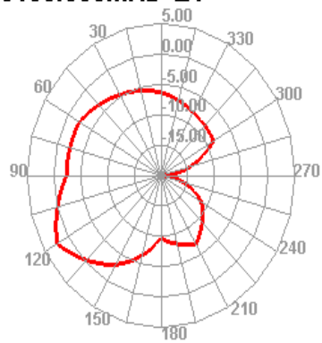
5150.000MHz E1
