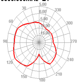
5550.000MHz E1
