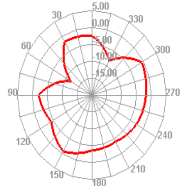
5850.000MHz E2
