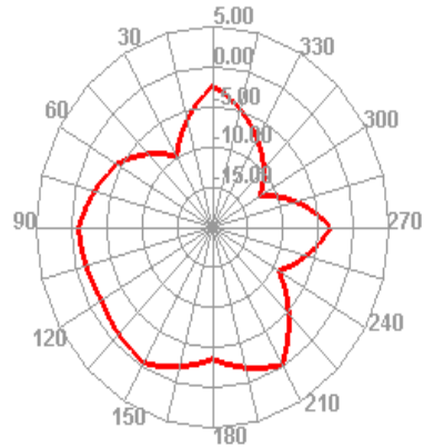
5850.000MHz E1
