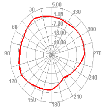
5850.000MHz H
