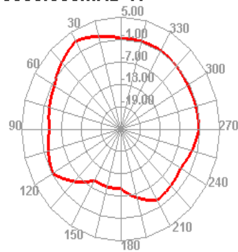
5550.000MHz H
