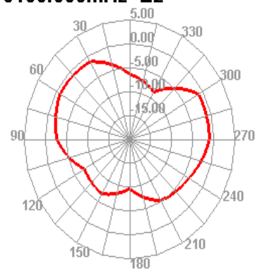
5150.000MHz E2
