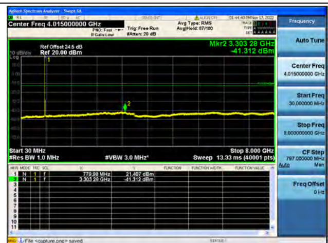
Band13 / 5MHz / Mid CH / 64QAM
