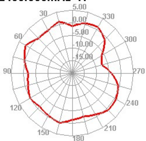
2430.000MHz E2
