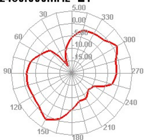
2440.000MHz
