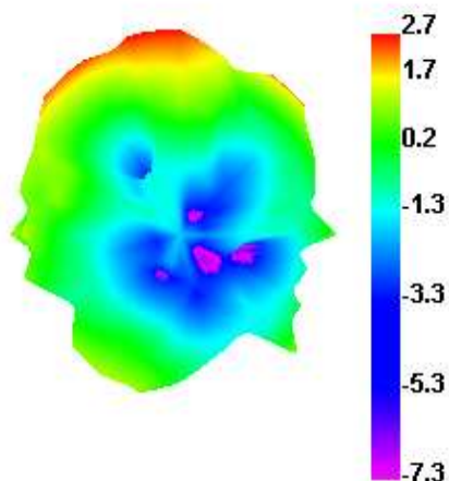
2490.000MHz E1
