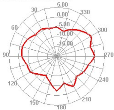
2450.000MHz E1
