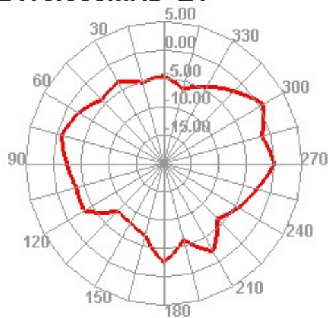
2470.000MHz
