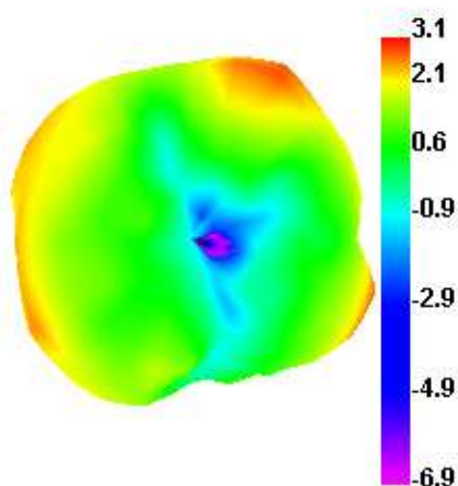
2480.000MHz E1
