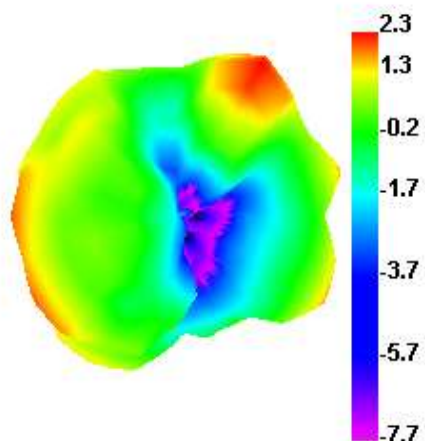
2430.000MHz E1
