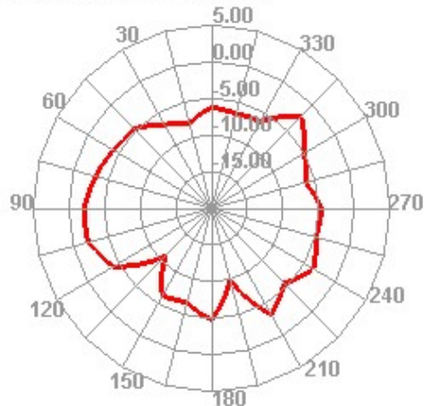
2450.000MHz H
