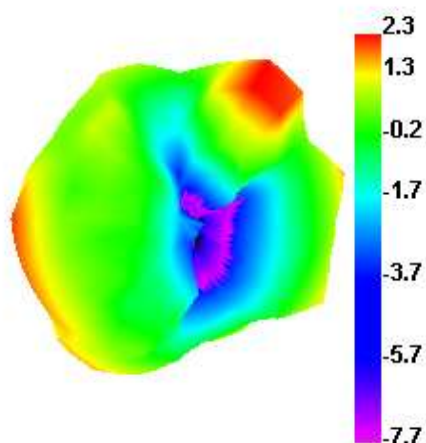
2400.000MHz E1
