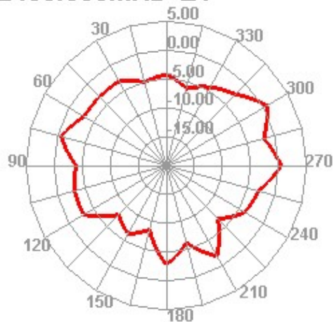
2480.000MHz E1
