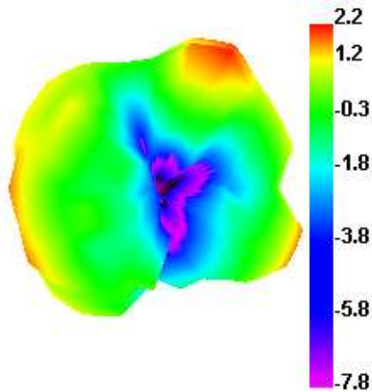
2460.000MHz E1
