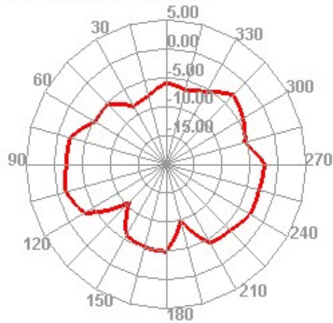
2420.000MHz H
