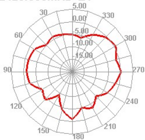
2420.000MHz E1
