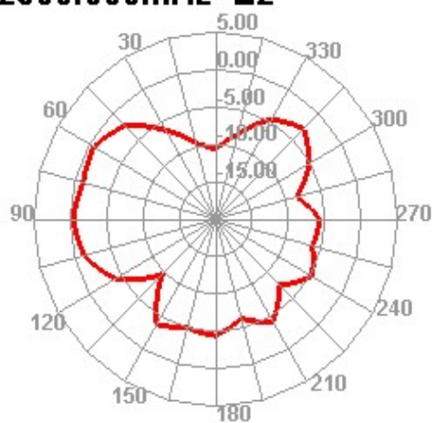
2500.000MHz E2
