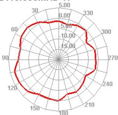
2410.000MHz H
