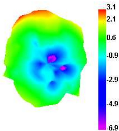
2450.000MHz E1
