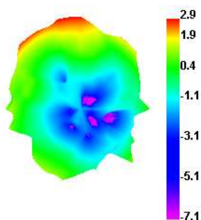
2480.000MHz E1
