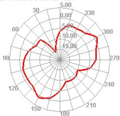
2450.000MHz E1
