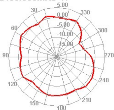
2400.000MHz H
