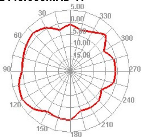
2440.000MHz H
