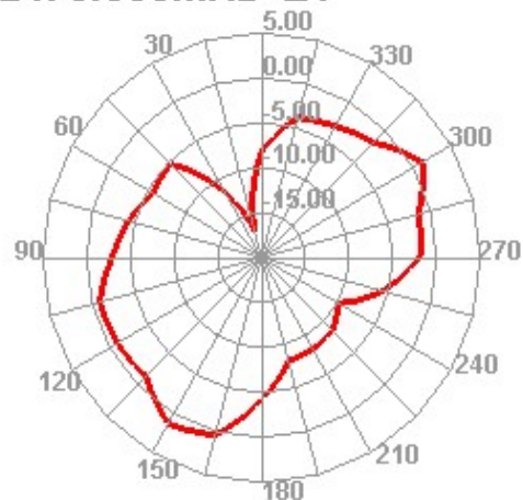
2480.000MHz
