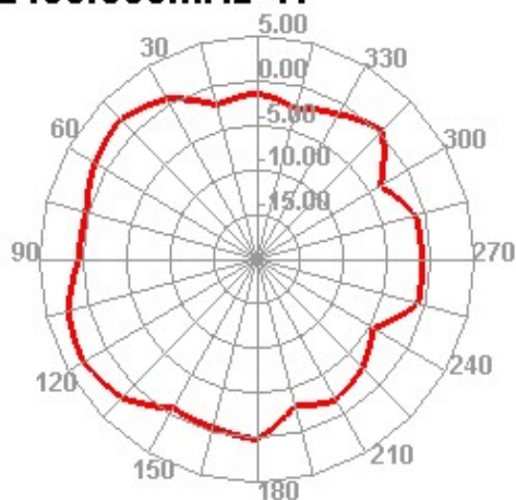
2430.000MHz E2
