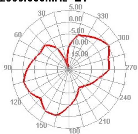
2500.000MHz E1
