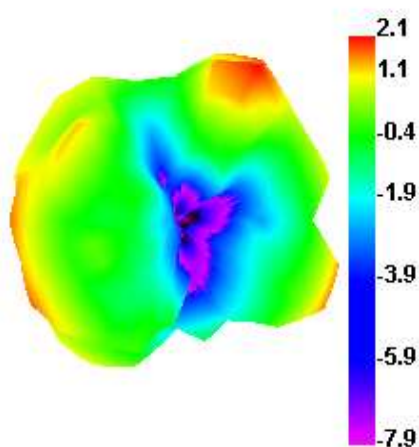
2450.000MHz E1
