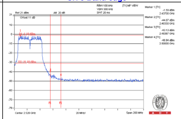
CH 9 Band edge
