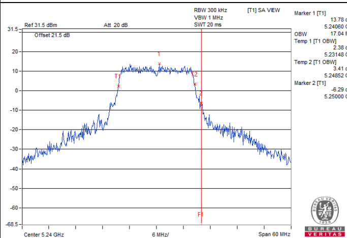
802.11a / Chain 3 : CH 48
