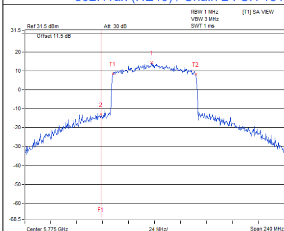
802.11ax (HE80) / Chain 1 : CH 155
