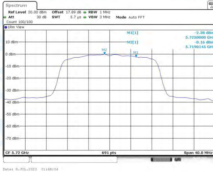
11AC20-CDD_Ant1_5720_UNII-3
