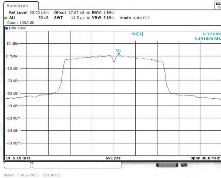
11N40-CDD_Ant2_5190
