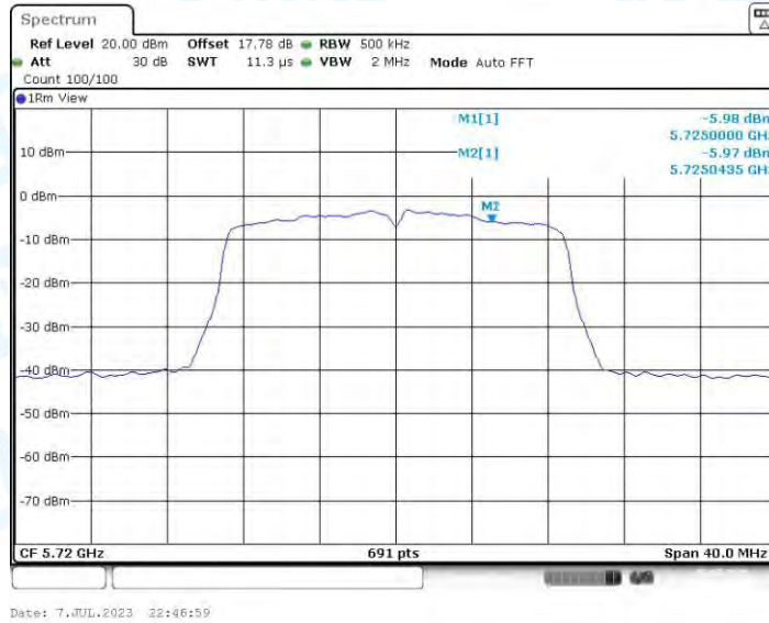
11N20-CDD_Ant3_5720_UNII-3
