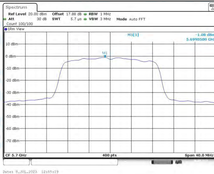
11N20-BF_Ant2_5700
