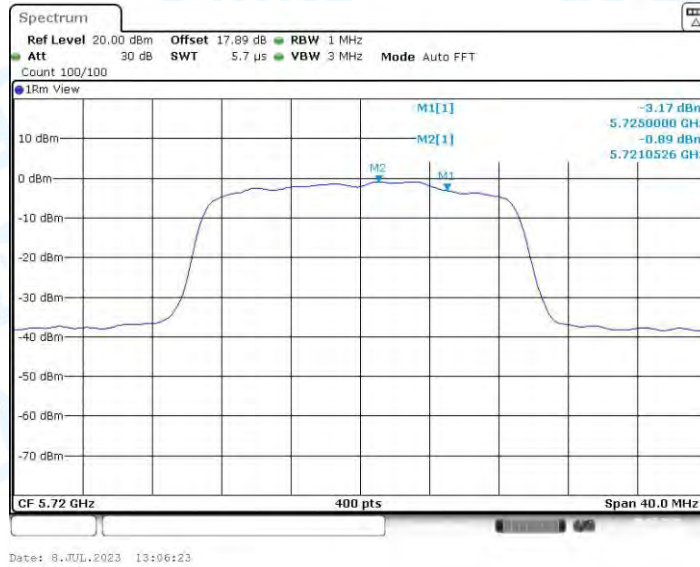
11N20-BF_Ant1_5720_UNII-3
