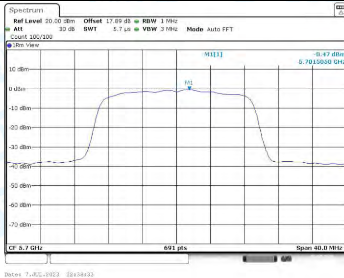
11N20-CDD_Ant3_5700
