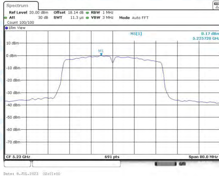
11AC40-CDD_Ant3_5230
