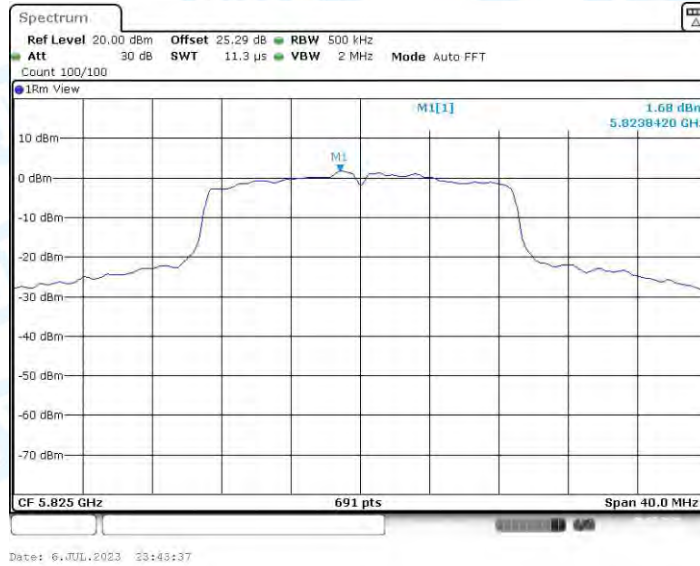
11N20-BF_Ant2_5825
