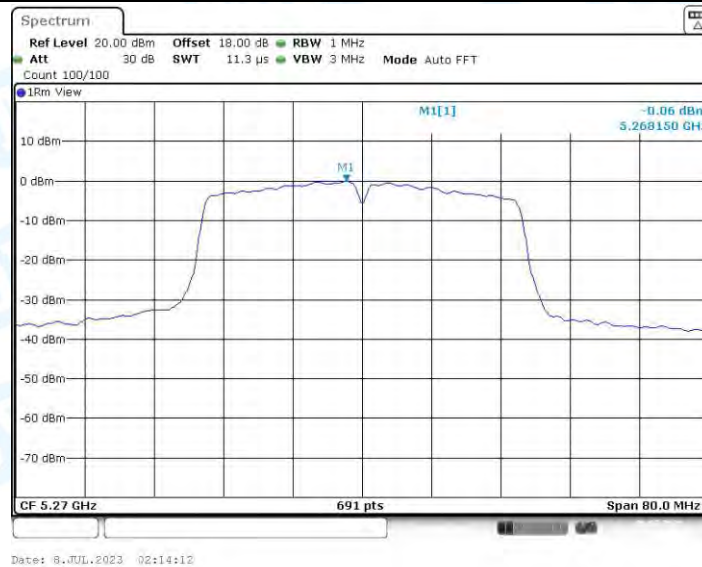
11AC40-CDD_Ant2_5270
