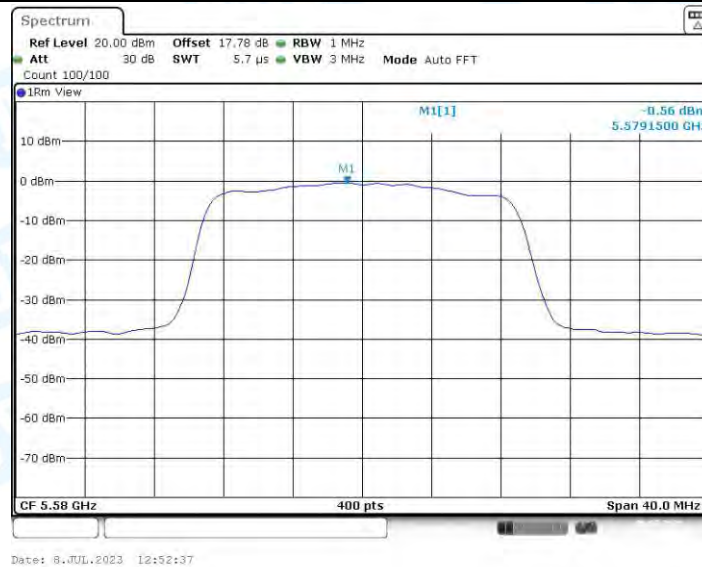
11N20-BF_Ant2_5580
