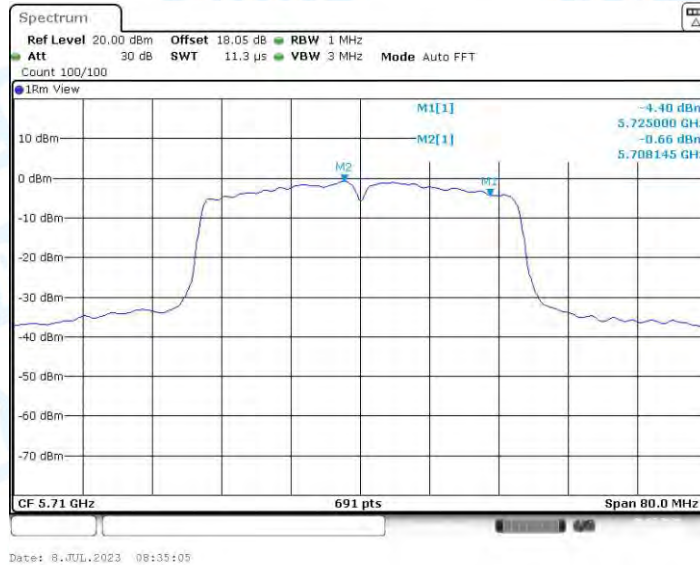
11AC40-CDD_Ant1_5710_UNII-3
