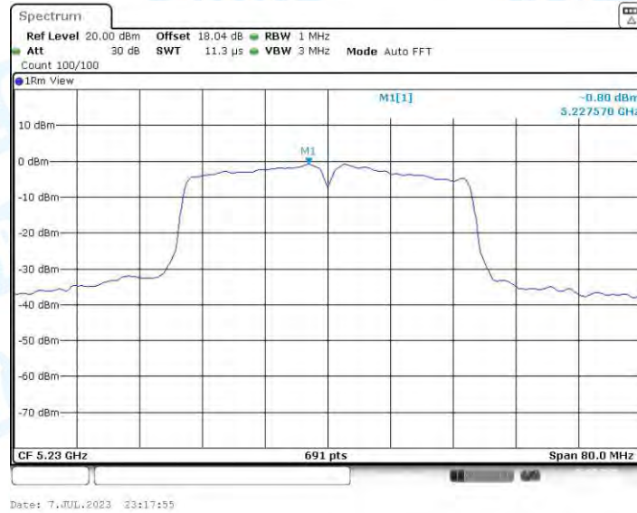
11N40-CDD_Ant4_5230
