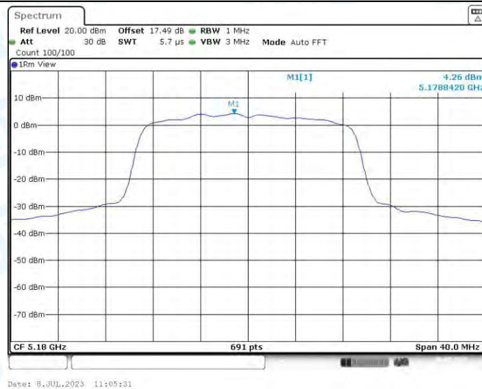
11N20-BF_Ant3_5180
