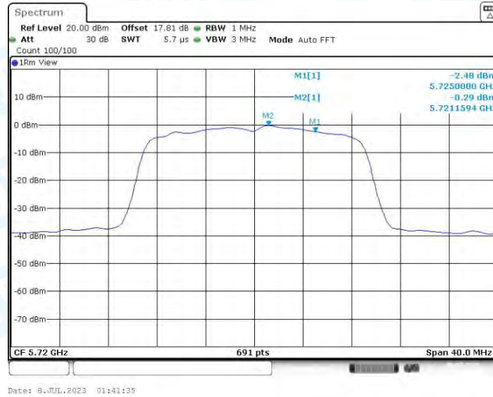
11AC20-CDD_Ant3_5720_UNII-2C
