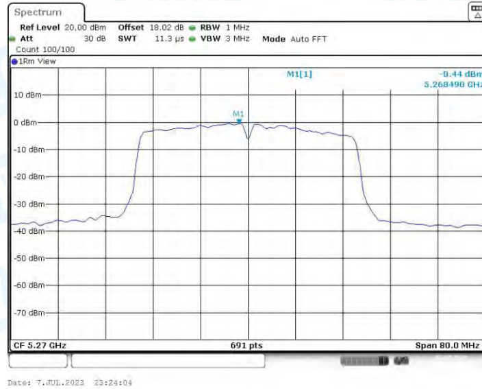
11N40-CDD_Ant3_5270
