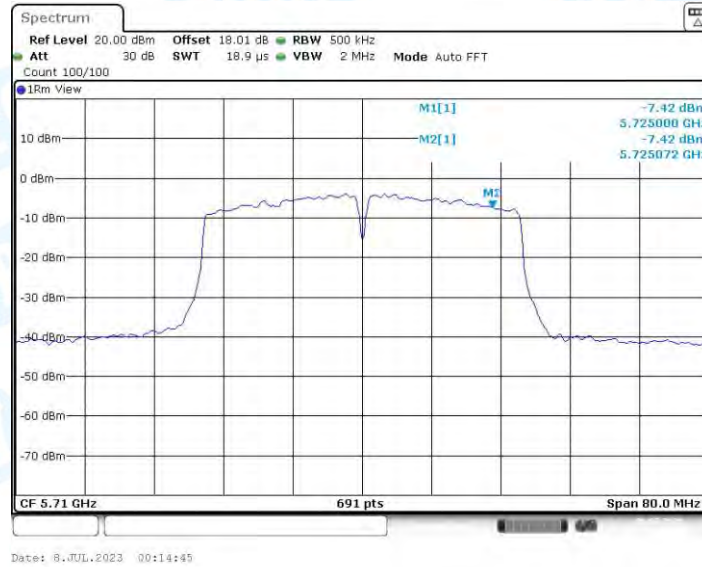
11N40-CDD_Ant3_5710_UNII-3
