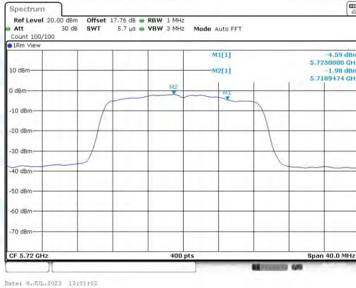
11N20-BF_Ant2_5720_UNII-2C
