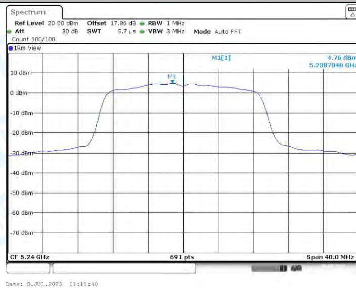
11N20-BF_Ant2_5240
