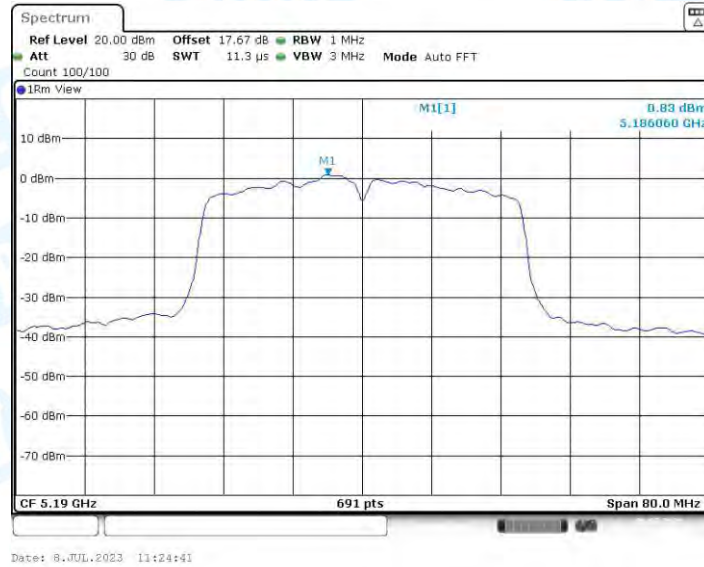
11N40-BF_Ant3_5190
