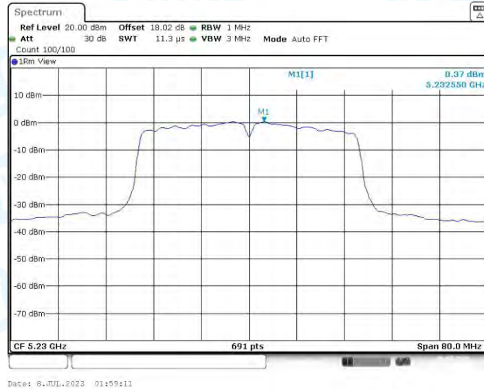
11AC40-CDD_Ant2_5230
