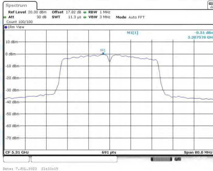
11N40-CDD_Ant3_5310
