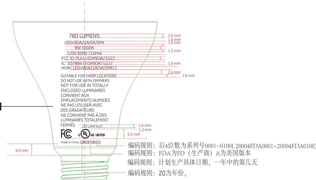
LED灯9W 5000K 版本（背面）
