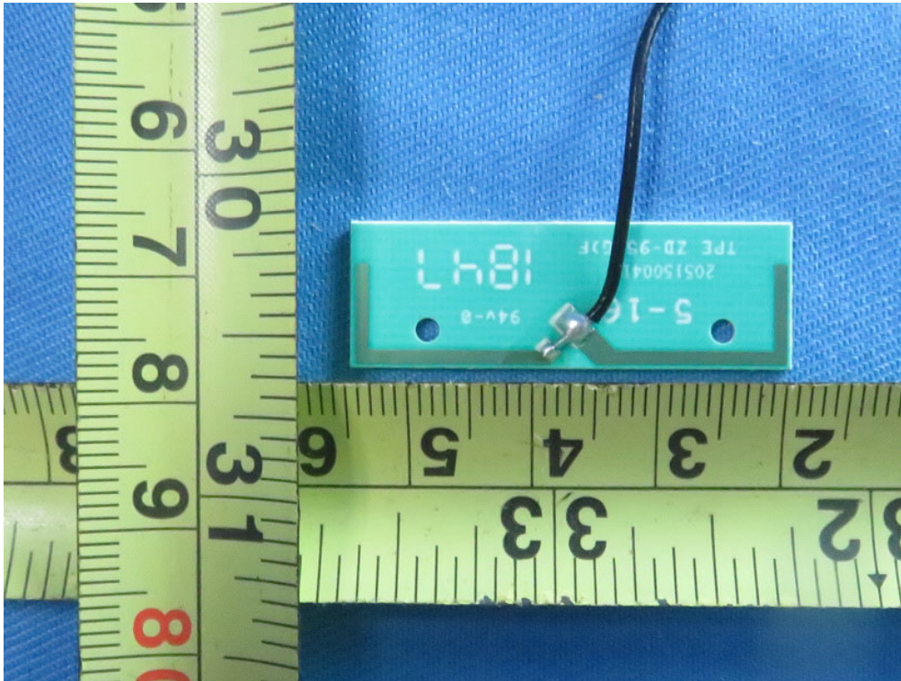
2.4GHz Ant.2
