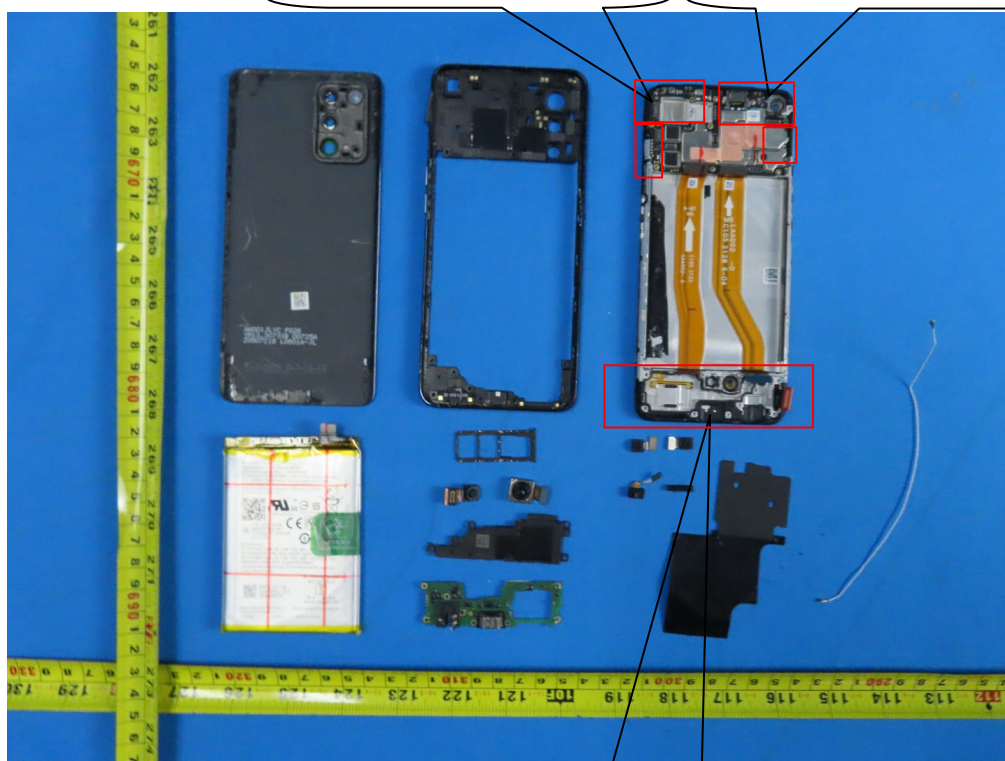
BT/WIFI/GPS Antenna
