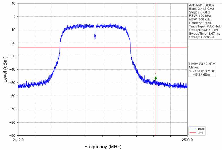
802.11n(HT40)_HCH_2452MHz_Ant1 (SISO)_NTNV
