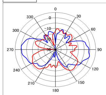
3700MHz Red:Vertical
