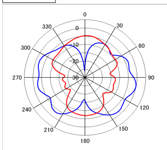
1710MHz(B4/B66) Red:Vertical
