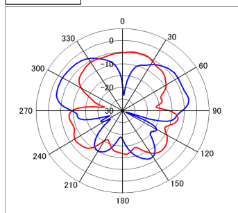
2500MHz Red:Vertical
