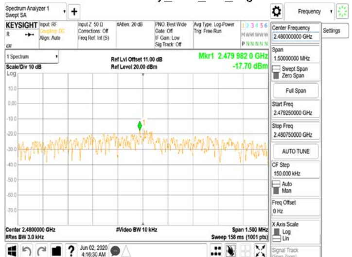
BLE 2M\Power Density_BLE_2M_HighCH39-2480
