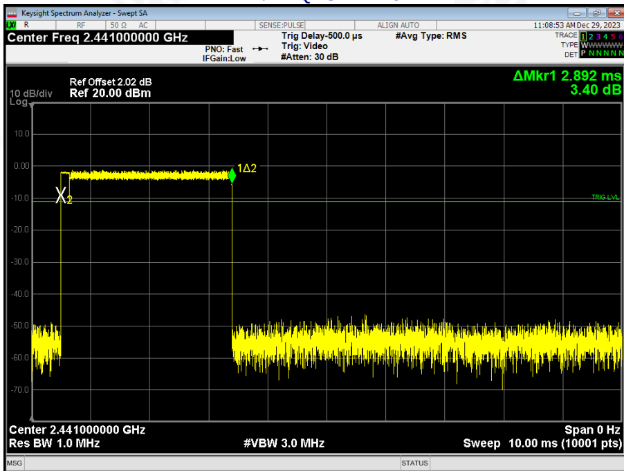
\pi/4 -DQPSK 2DH5 2441MHz
