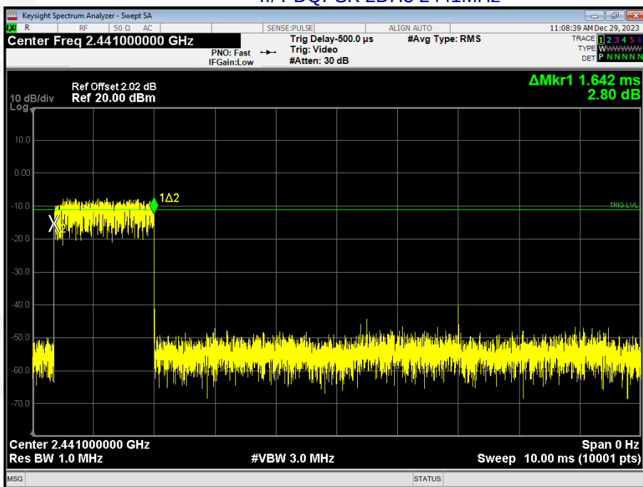
\pi/4 -DQPSK 2DH3 2441MHz
