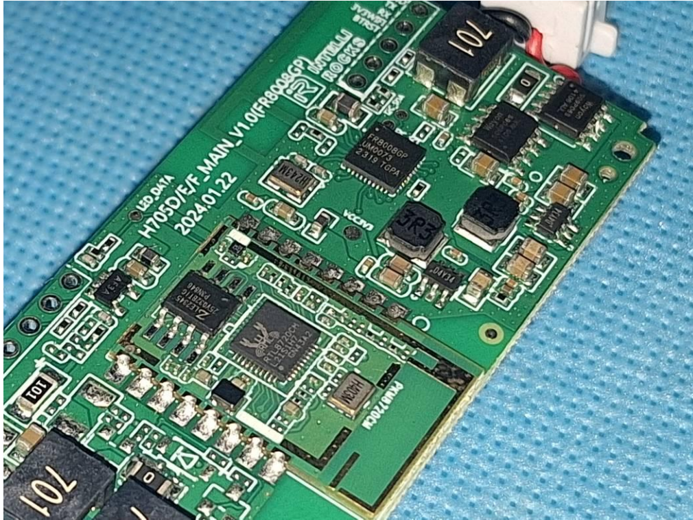
Model: H705F
