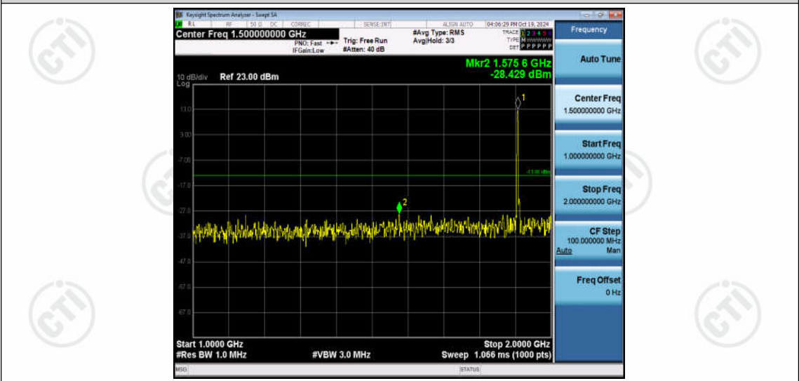
Band2-5MHz-16QAM-19175-1RB#0-Range2:1000~2000MHz
