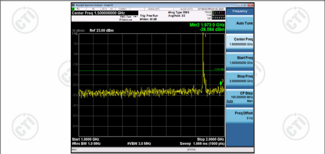
Band2-20MHz-16QAM-19100-1RB#0-Range2:1000~2000MHz
