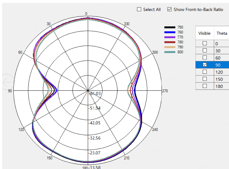
B13 Phi=90deg
