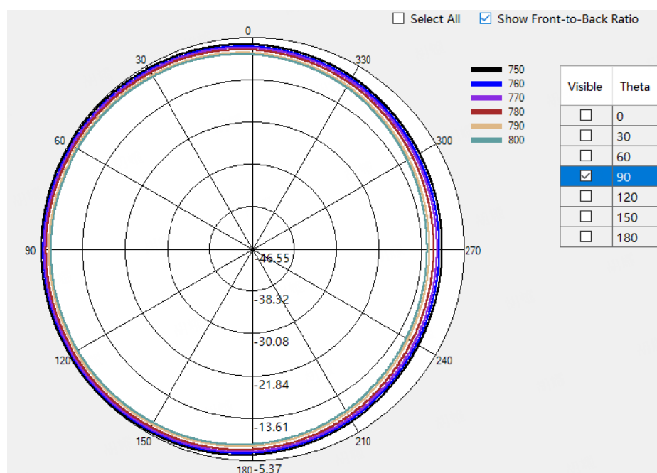
B13 Theta=90deg
