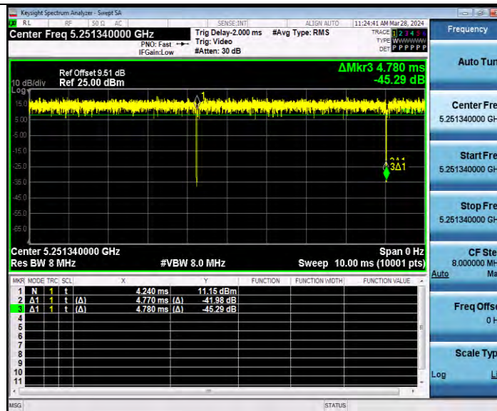
11AX20MIMO_Ant2_5260_26Tone_RU0
