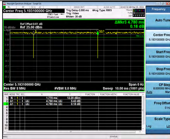
11AX20MIMO_Ant2_5200_26Tone_RU4
