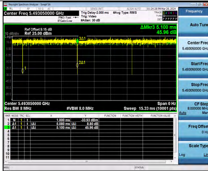
11AX20MIMO_Ant2_5500_26Tone_RU0
