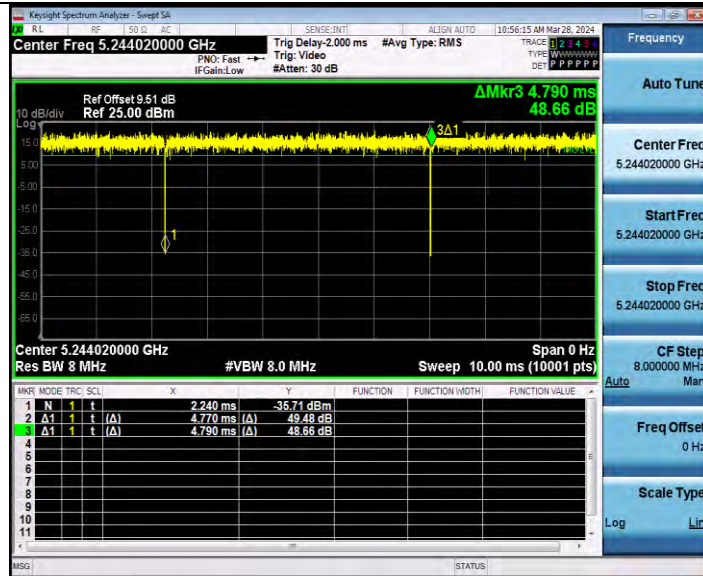
11AX20MIMO_Ant2_5240_26Tone_RU8
