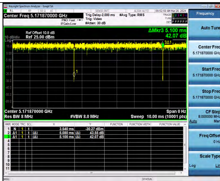
11AX20MIMO_Ant2_5180_106Tone_RU53
