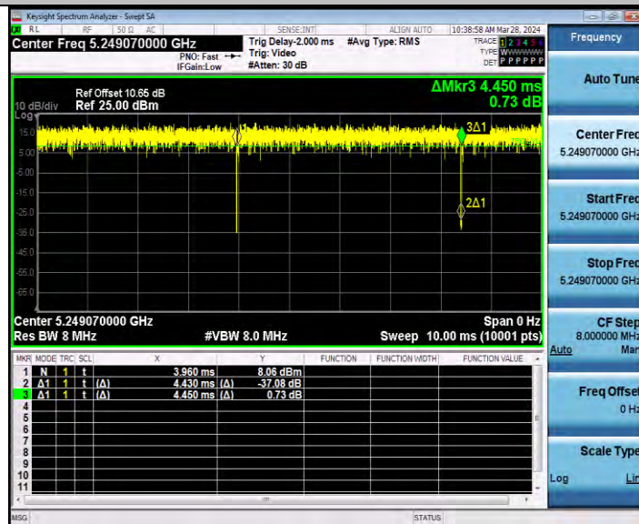
11AX20MIMO_Ant2_5240_52Tone_RU40
