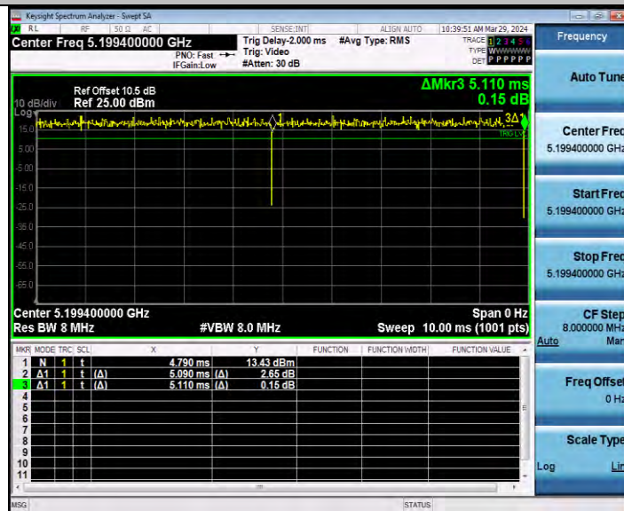
11AX20MIMO_Ant2_5200_52Tone_RU38
