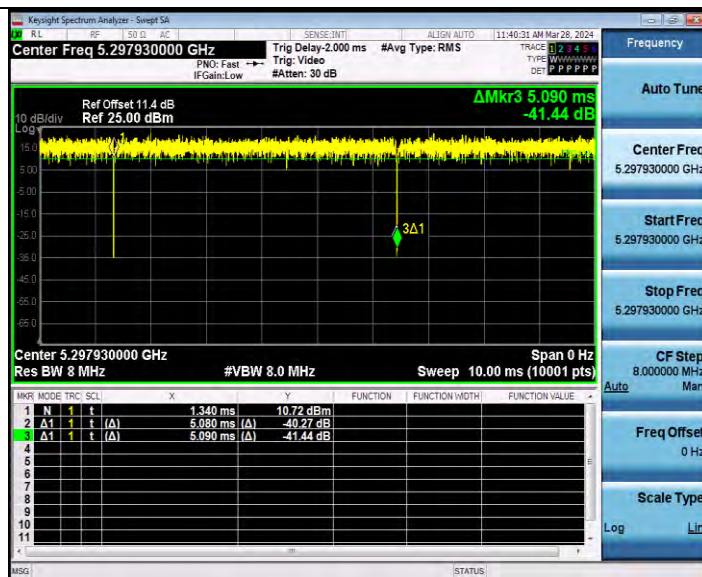
11AX20MIMO_Ant2_5300_106Tone_RU53
