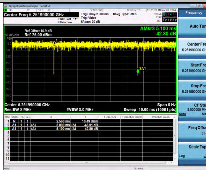
11AX20MIMO_Ant2_5260_52Tone_RU37
