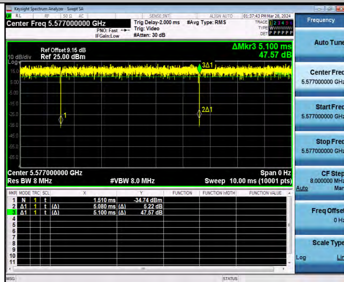
11AX20MIMO_Ant1_5580_106Tone_RU53
