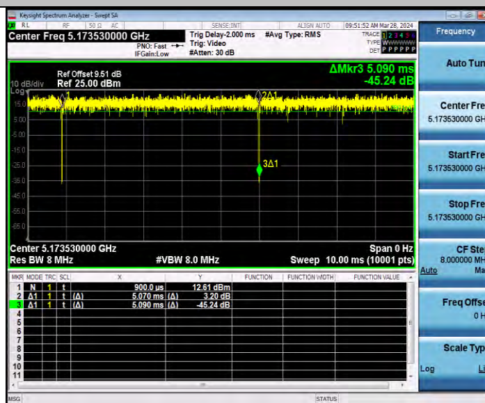
11AX20MIMO_Ant1_5180_106Tone_RU53
