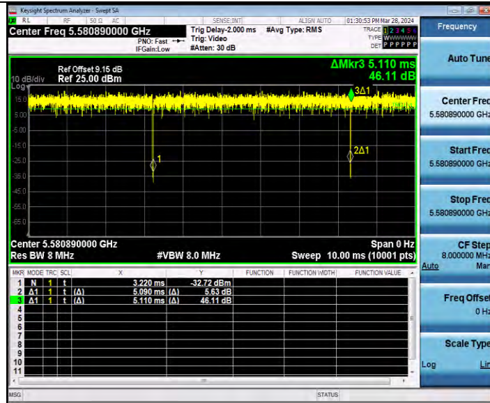
11AX20MIMO_Ant1_5580_52Tone_RU38
