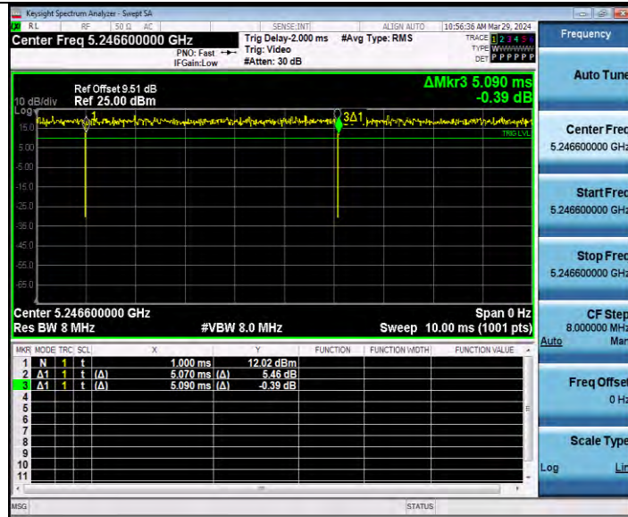
11AX20MIMO_Ant1_5240_52Tone_RU40
