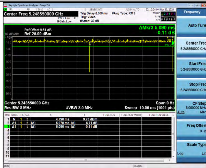
11AX20MIMO_Ant1_5240_106Tone_RU54
