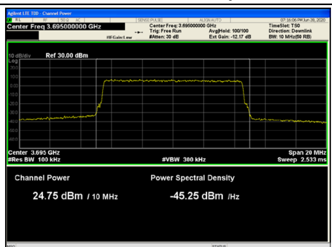
10MHz - Middle CH 64QAM
