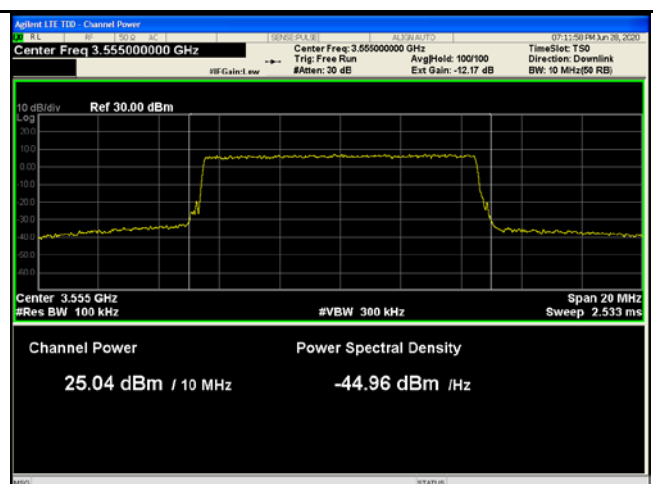
10MHz - Low CH 64QAM
