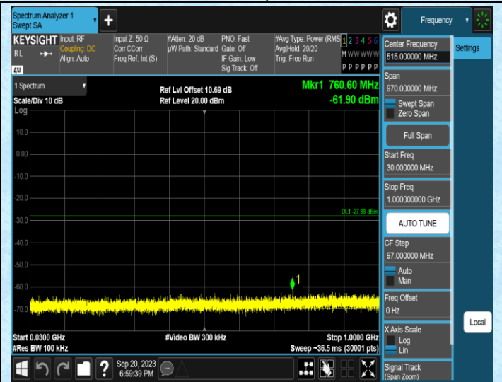
11N20MIMO-Ant0-2462-30~1000
