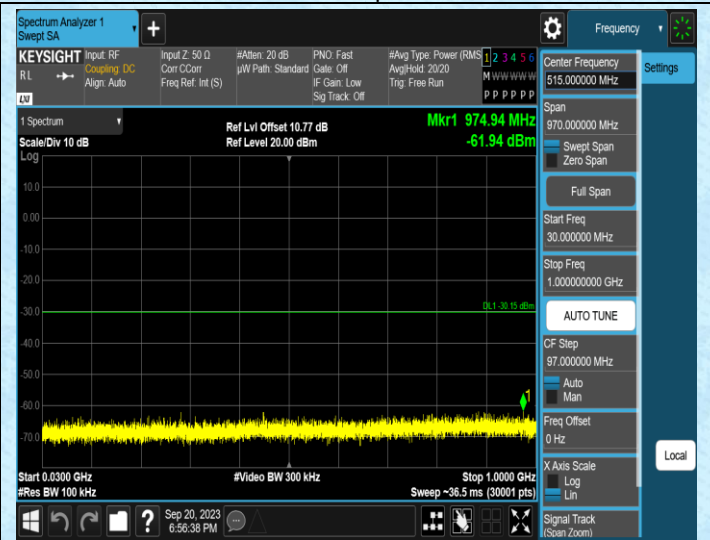
11N20MIMO-Ant0-2437-30~1000
