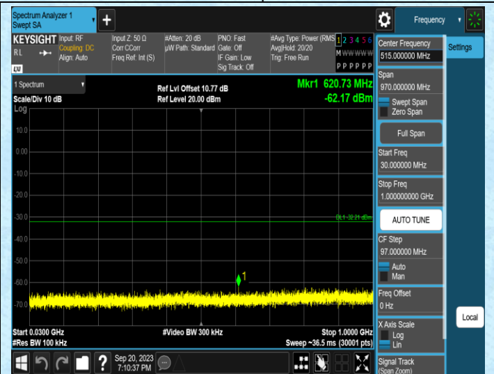
11N40MIMO-Ant0-2437-30~1000
