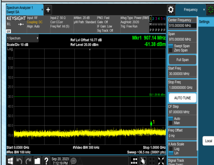
11N40MIMO-Ant1-2437-30~1000
