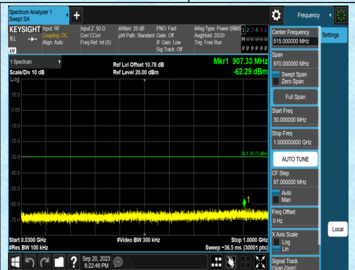
11N40SISO-Ant0-2422-30~1000
