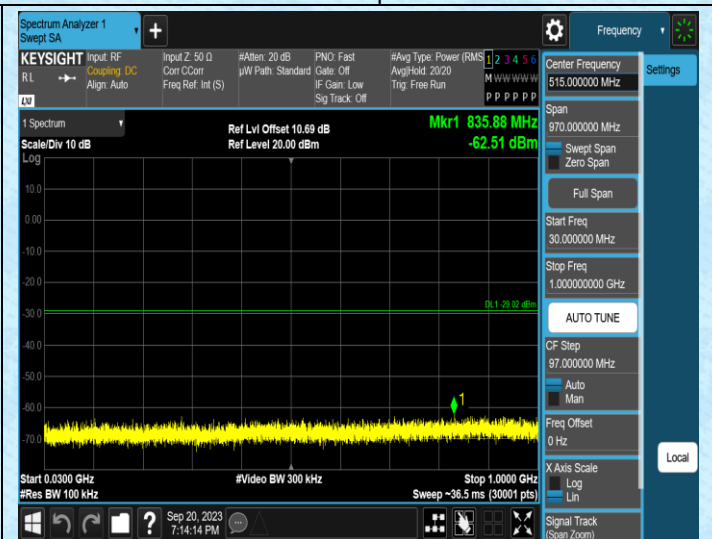
11N40MIMO-Ant0-2452-30~1000
