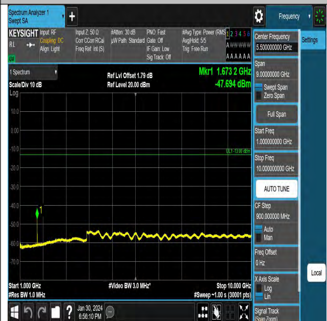
EGPRS850-190-8-1000~10000MHz-PASS
