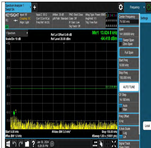
GSM850-190-5-0.009~0.15MHz-PASS
