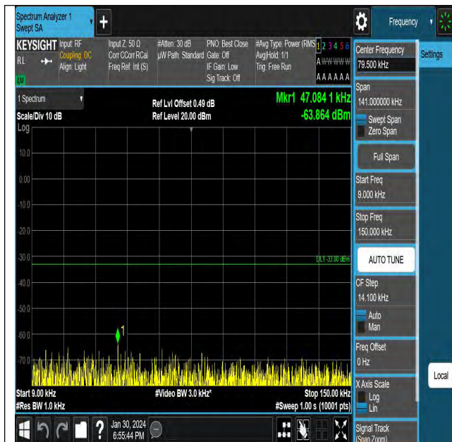
EGPRS850-190-8-0.009~0.15MHz-PASS
