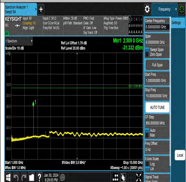
GSM850-190-5-1000~10000MHz-PASS
