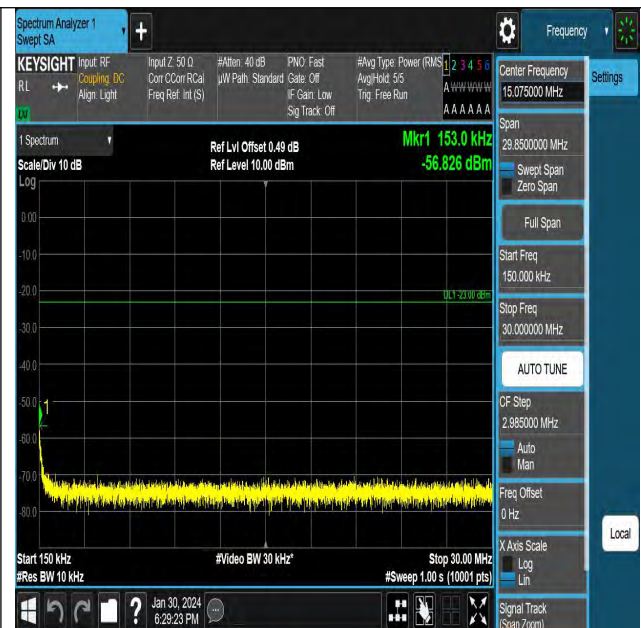
GSM850-251-5-0.15~30MHz-PASS
