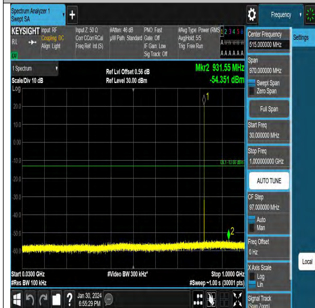
EGPRS850-128-8-30~1000MHz-PASS
