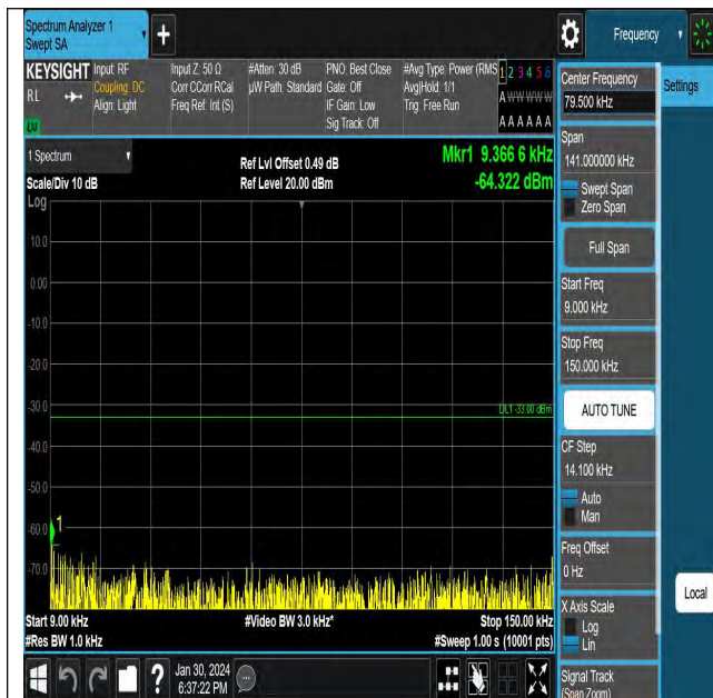
GPRS850-128-5-0.009~0.15MHz-PASS
