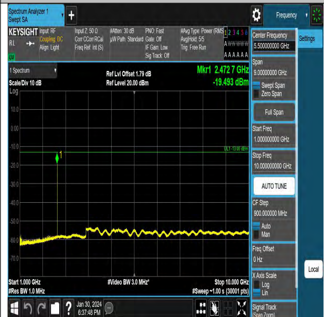
GPRS850-128-5-1000~10000MHz-PASS
