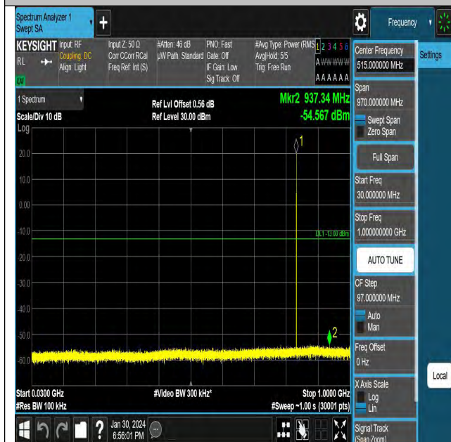
EGPRS850-190-8-30~1000MHz-PASS
