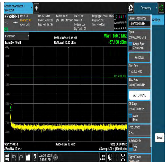
GPRS850-128-5-0.15~30MHz-PASS
