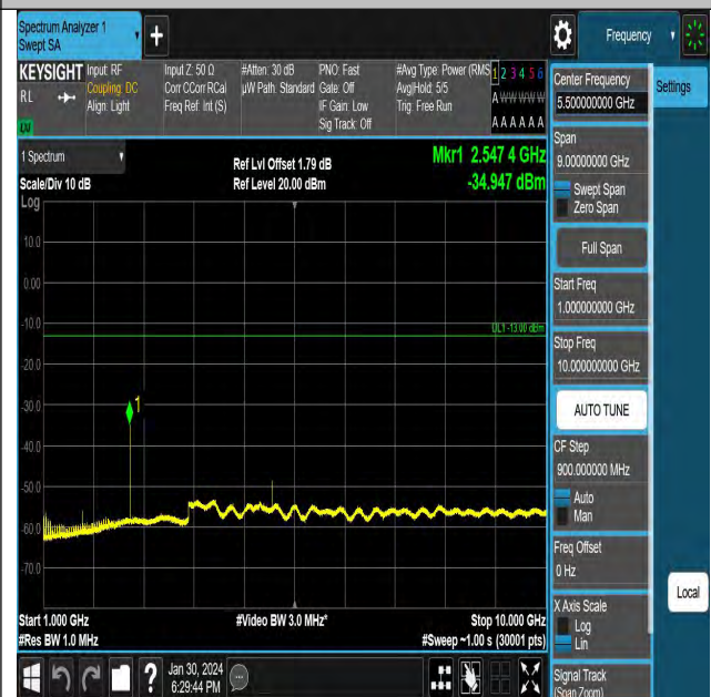
GSM850-251-5-1000~10000MHz-PASS
