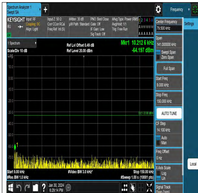
GSM850-251-5-0.009~0.15MHz-PASS
