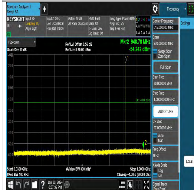
GPRS850-128-5-30~1000MHz-PASS
