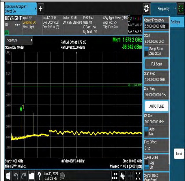
GPRS850-190-5-1000~10000MHz-PASS
