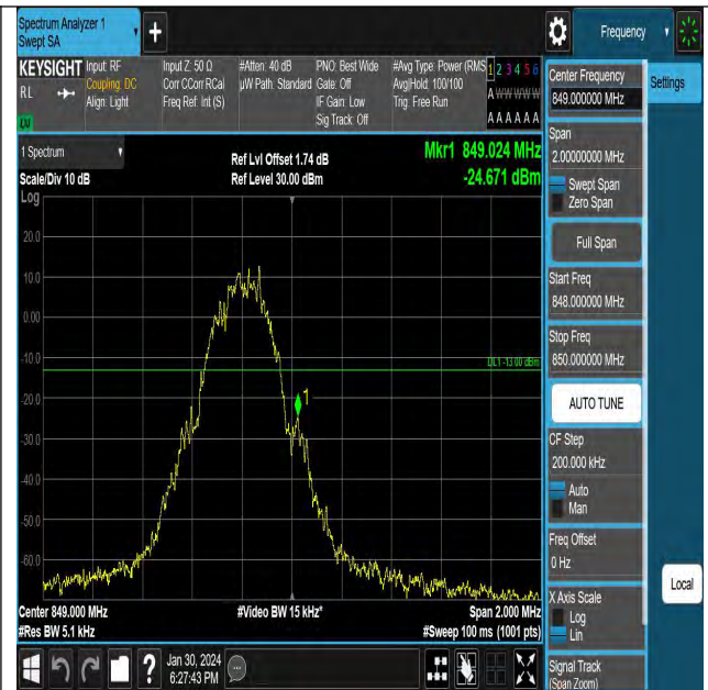
GSM850-251-5-PASS
