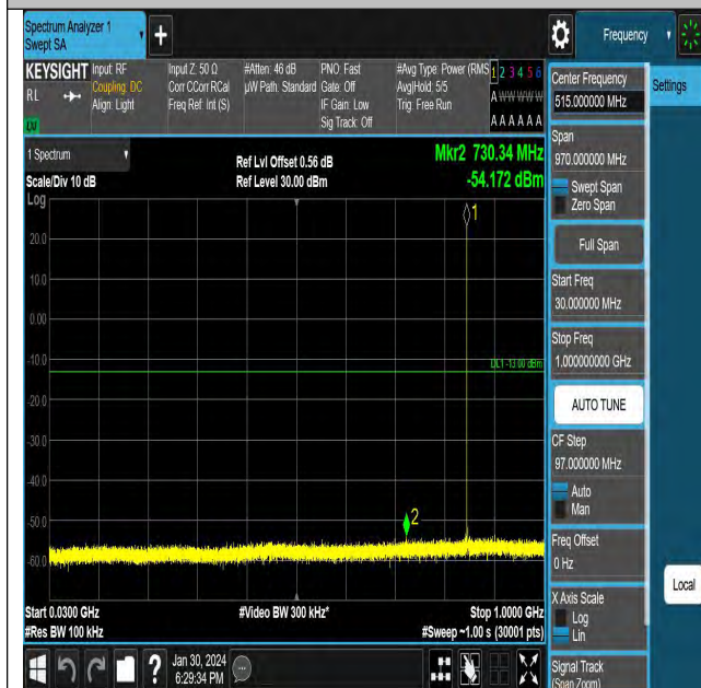
GSM850-251-5-30~1000MHz-PASS
