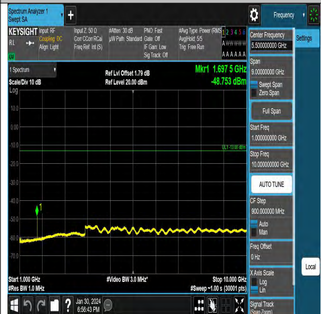
EGPRS850-251-8-1000~10000MHz-PASS
