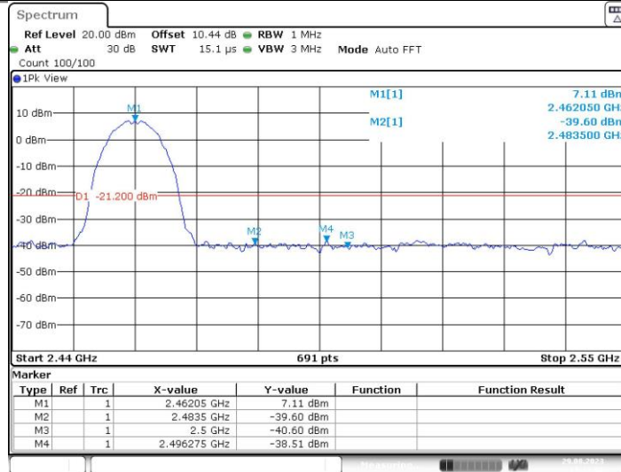
11G Ant1 Low 2412 AV
