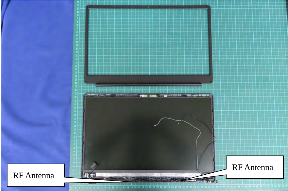
(30) EUT Photo
