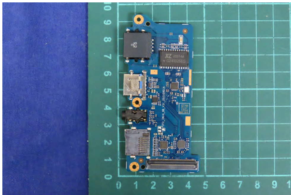
(16) EUT Photo
