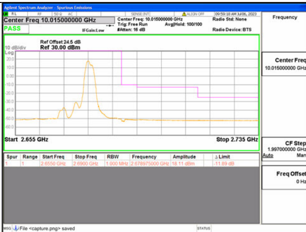
41C / 20+10MHz / High CH / QPSK / 1#99-1#0
