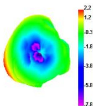
2500.000MHz
