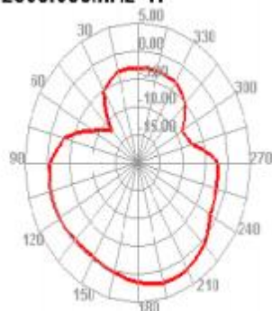
2500.000MHz H
