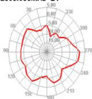
2500.000MHz E1
