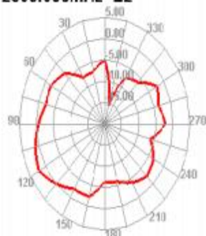
2500.000MHz E2
