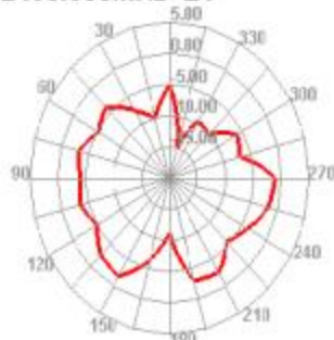
2450.000MHz E1
