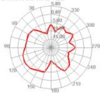
2400.000MHz E2
