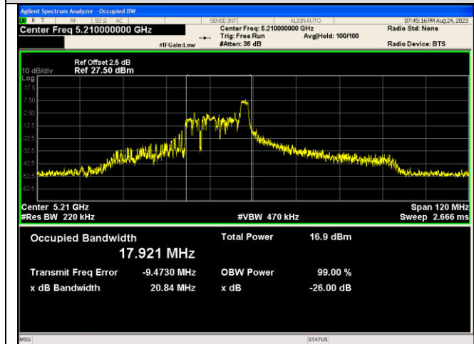
IEEE 802.11ax_Channel 42_80MHz_Antenna 0_RU&amp;Index 26RU17
