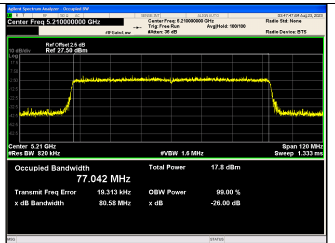
IEEE 802.11ax_Channel 42_80MHz_Antenna 1_RU&amp;Index 996RU67
