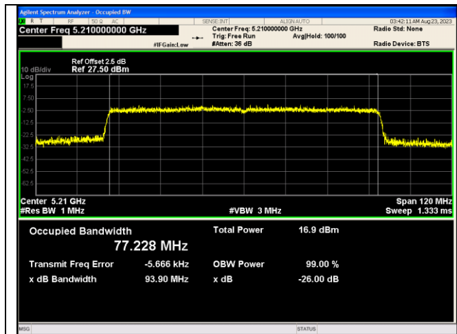
IEEE 802.11ax_Channel 42_80MHz_Antenna 0_RU&amp;Index 996RU67
