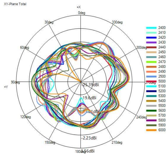
(3)X-Y Plane(unit:dBi):
