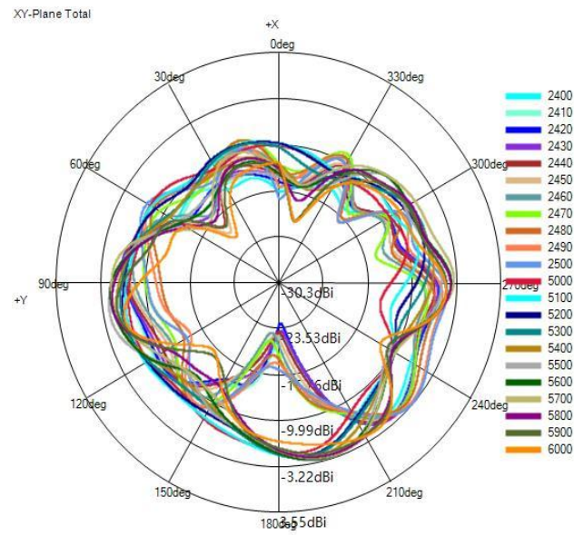
(3)X-Y Plane(unit:dBi):
