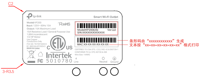
尺寸图 (54.00*29.00mm)
