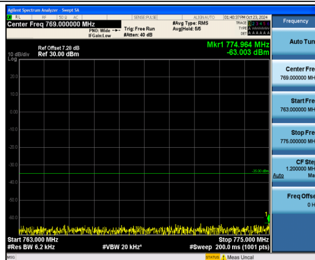
Band13-5MHz-16QAM-23230-1-0-Low-763-775--63-PASS
