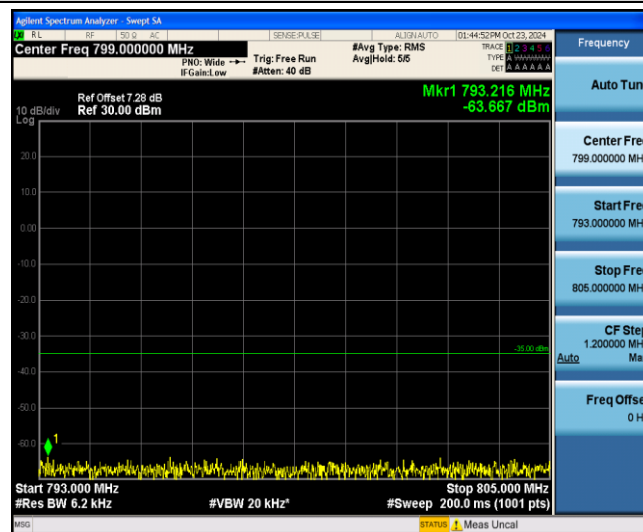
Band13-5MHz-16QAM-23255-1-0-Low-793-805--63.67-PASS
