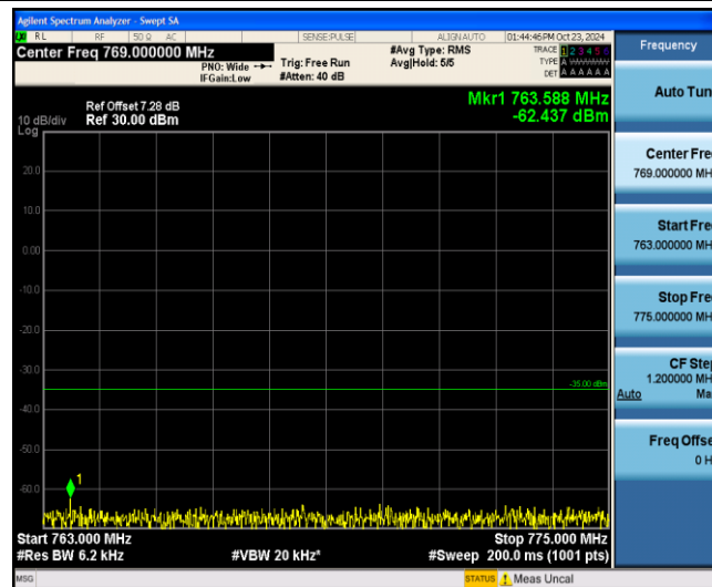
Band13-5MHz-16QAM-23255-1-0-Low-763-775--62.44-PASS
