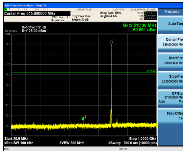
Band12-10MHz-QPSK-23060-1-0-Low-30-1000--60.85-PASS
