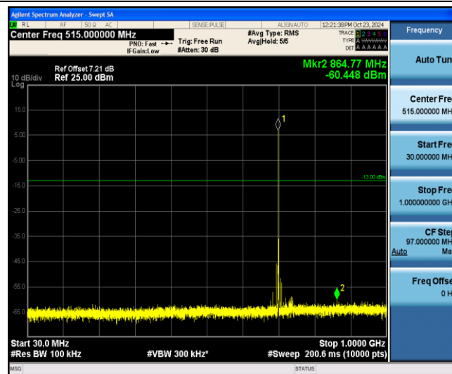
Band12-10MHz-QPSK-23130-1-0-Low-30-1000--60.45-PASS
