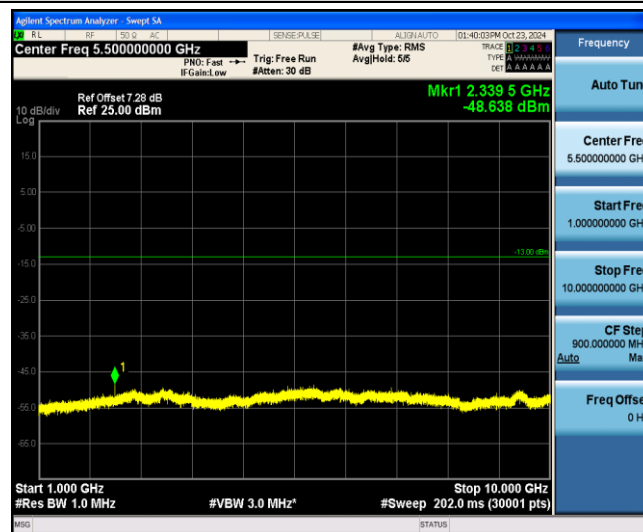
Band13-5MHz-QPSK-23230-1-0-Low-1000-10000--48.64-PASS
