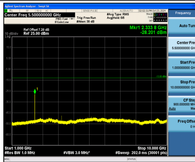
Band13-10MHz-16QAM-23230-1-0-Low-1000-10000--28.2-PASS
