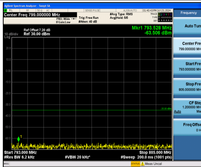
Band13-5MHz-16QAM-23230-1-0-Low-793-805--63.51-PASS
