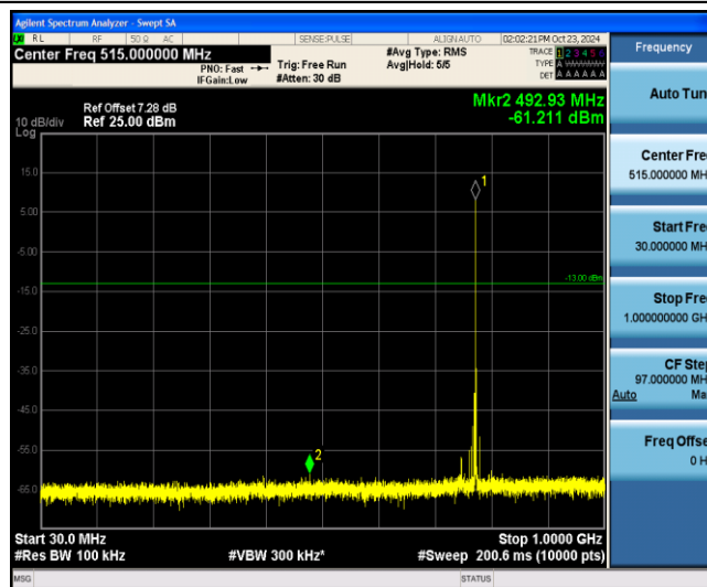
Band13-10MHz-16QAM-23230-1-0-Low-30-1000--61.21-PASS
