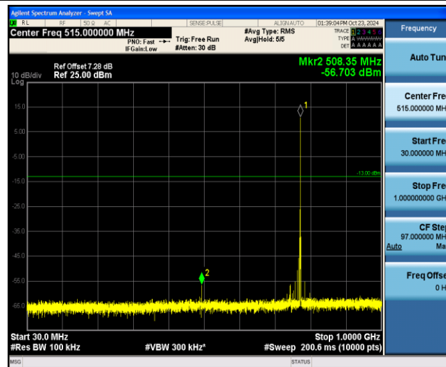
Band13-5MHz-16QAM-23205-1-0-Low-30-1000--56.7-PASS
