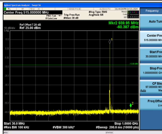
Band13-5MHz-QPSK-23255-1-0-Low-30-1000--60.39-PASS
