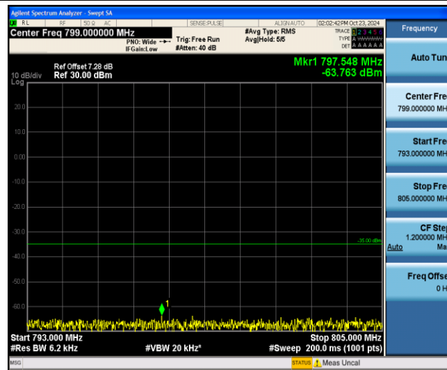
Band13-10MHz-16QAM-23230-1-0-Low-793-805--63.76-PASS
