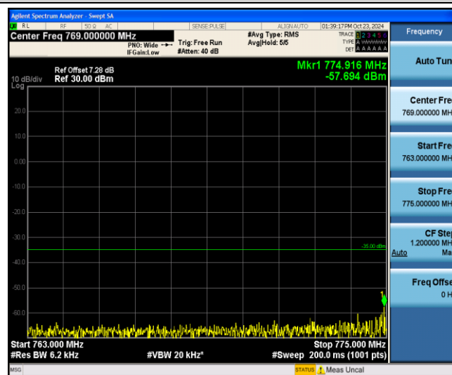
Band13-5MHz-16QAM-23205-1-0-Low-763-775--57.69-PASS
