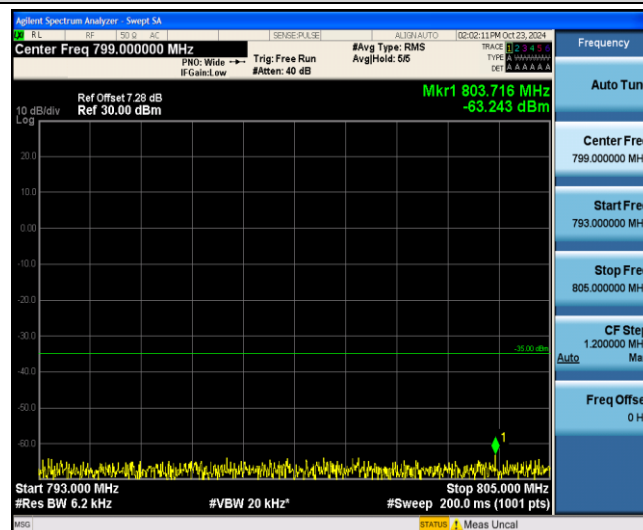
Band13-10MHz-QPSK-23230-1-0-Low-793-805--63.24-PASS
