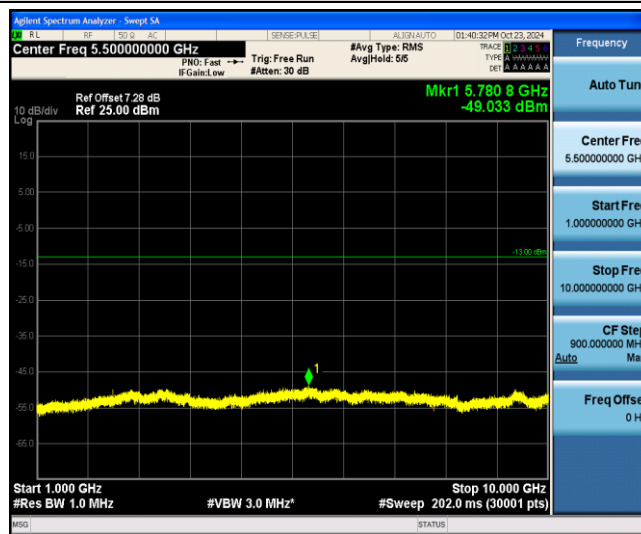
Band13-5MHz-16QAM-23230-1-0-Low-1000-10000--49.03-PASS
