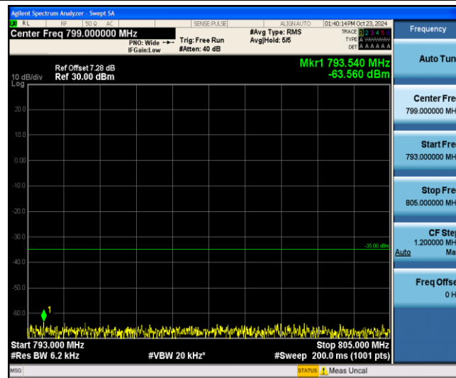
Band13-5MHz-QPSK-23230-1-0-Low-793-805--63.56-PASS
