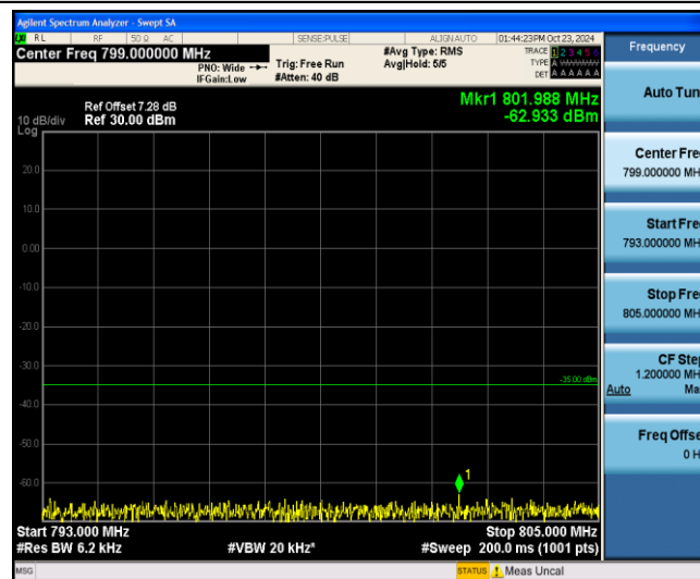
Band13-5MHz-QPSK-23255-1-0-Low-793-805--62.93-PASS
