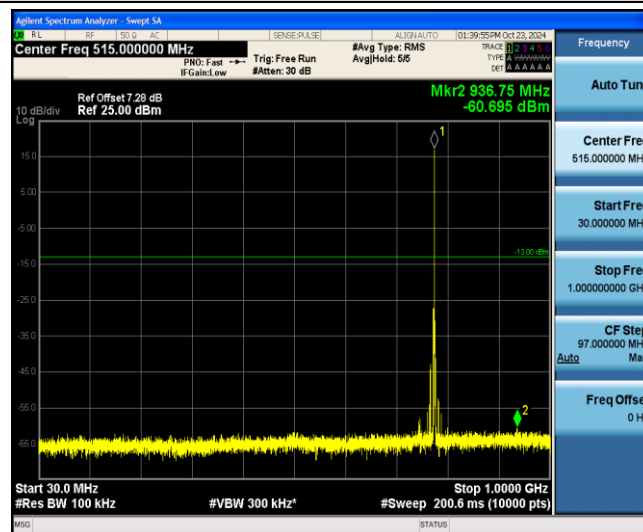
Band13-5MHz-QPSK-23230-1-0-Low-30-1000--60.7-PASS
