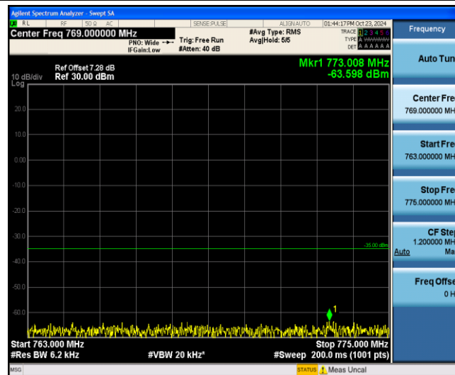
Band13-5MHz-QPSK-23255-1-0-Low-763-775--63.6-PASS
