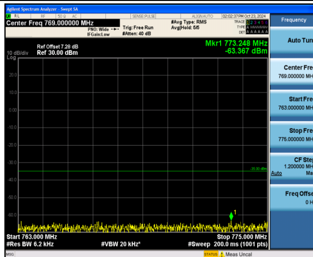
Band13-10MHz-16QAM-23230-1-0-Low-763-775--63.37-PASS
