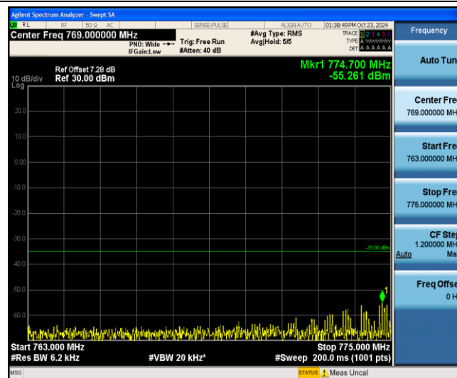
Band13-5MHz-QPSK-23205-1-0-Low-763-775--55.26-PASS
