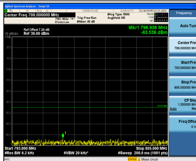
Band13-5MHz-QPSK-23205-1-0-Low-793-805--63.54-PASS
