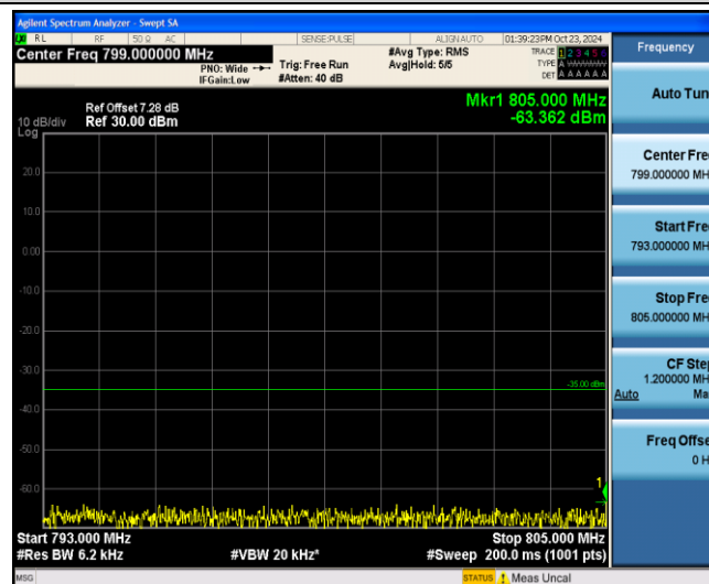
Band13-5MHz-16QAM-23205-1-0-Low-793-805--63.36-PASS
