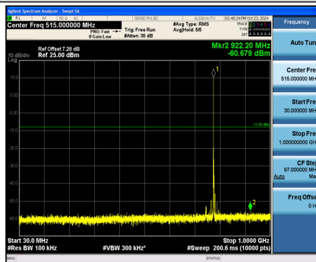
Band13-5MHz-16QAM-23230-1-0-Low-30-1000--60.68-PASS
