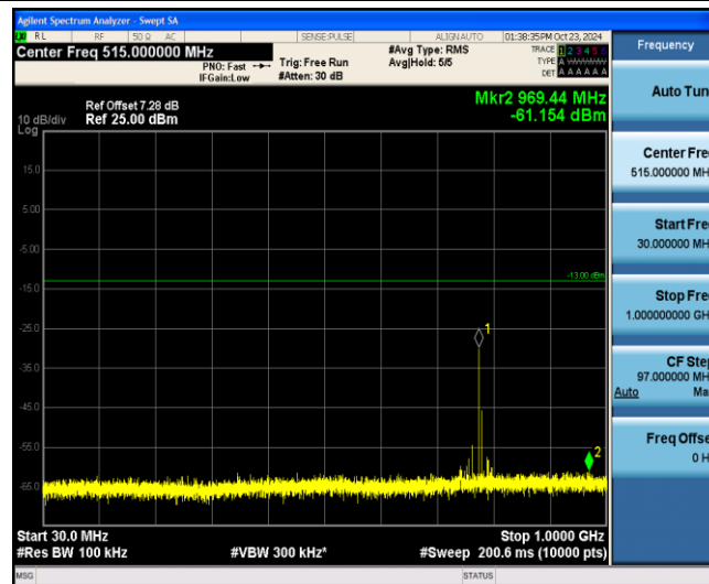
Band13-5MHz-QPSK-23205-1-0-Low-30-1000--61.15-PASS
