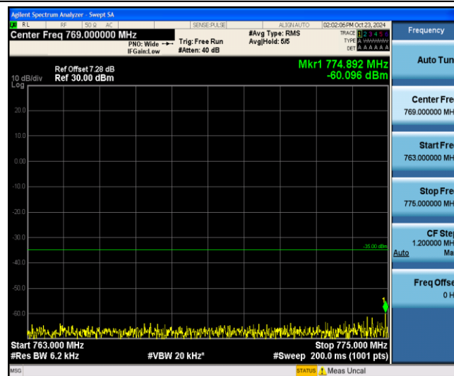
Band13-10MHz-QPSK-23230-1-0-Low-763-775--60.1-PASS
