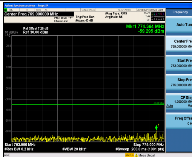
Band13-5MHz-QPSK-23230-1-0-Low-763-775--59.3-PASS
