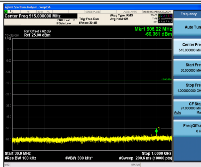
Band2-1.4MHz-QPSK-18900-1-0-Low-30-1000--60.35-PASS
