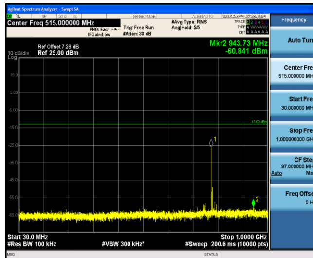
Band13-10MHz-QPSK-23230-1-0-Low-30-1000--60.84-PASS
