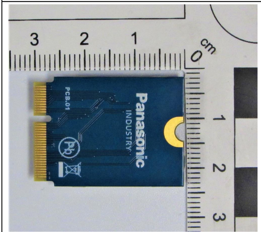
RF Module-PAN9019(A)-bottom
