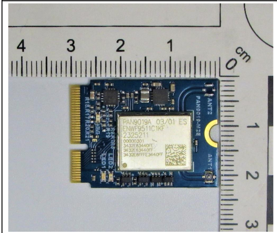
RF Module-PAN9019(A)-top
