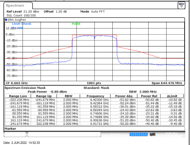
802.11ax (160MHz) /6665MHz / Chain D / NSS-4
