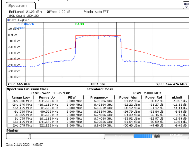
802.11ax (160MHz) /6665MHz / Chain C / NSS-4
