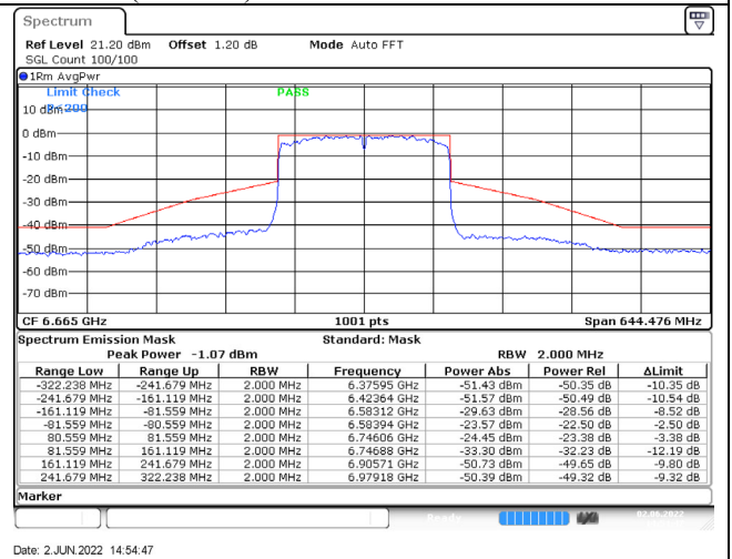
802.11ax (160MHz) /6665MHz / Chain B / NSS-4
