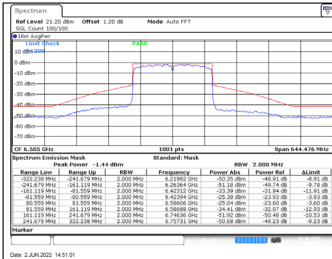
802.11ax (160MHz) /6505MHz / Chain C / NSS-4
