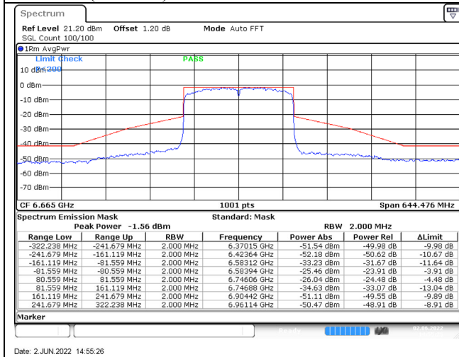
802.11ax (160MHz) /6665MHz / Chain A / NSS-4
