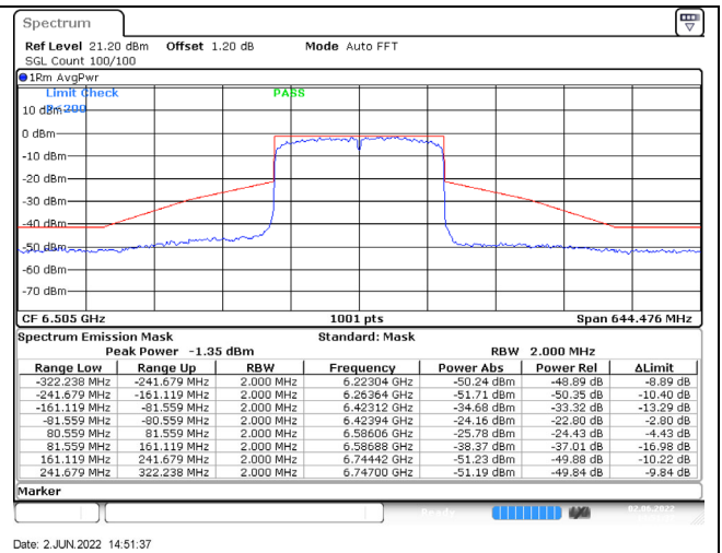
802.11ax (160MHz) /6505MHz / Chain D / NSS-4
