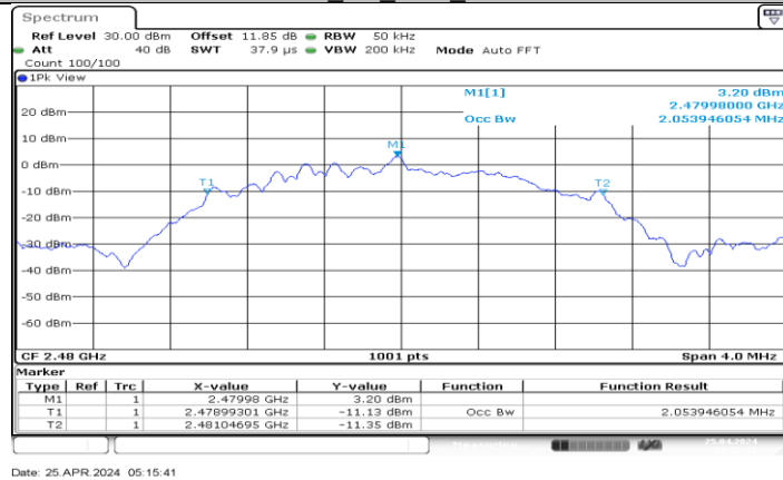
BLE_2M_Ant7_2480
