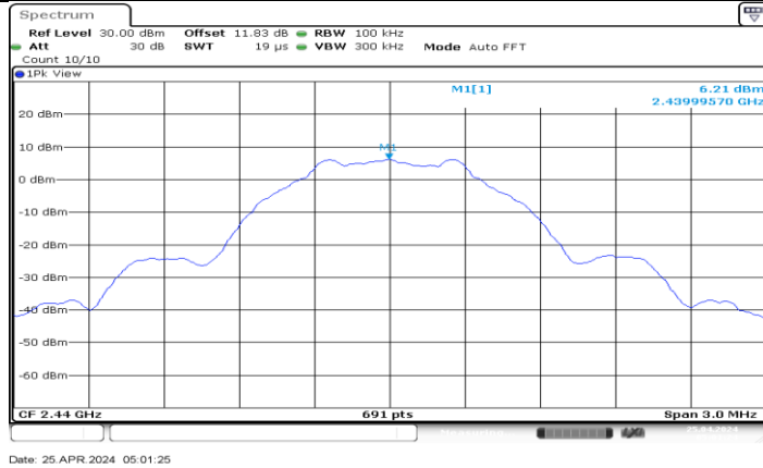
BLE 1M Ant7 2440 0-Reference
