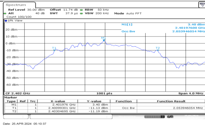
BLE_2M_Ant7_2402
