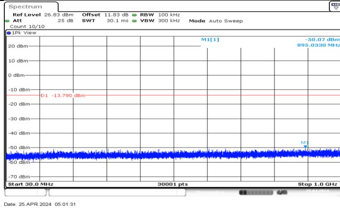
BLE 1M Ant7 2440 30-1000
