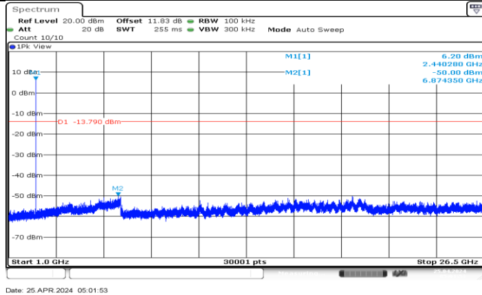
BLE 1M Ant7 2440 1000-26500
