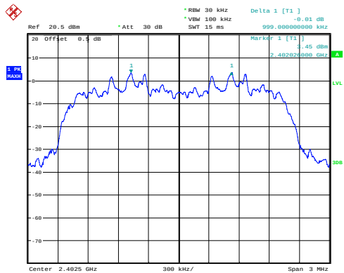
\pi/4 -DQPSK_Low 0.999MHz
