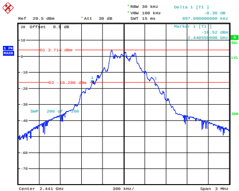
GFSK_Middle 0.897MHz
