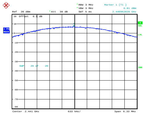
\pi/4 -DQPSK_Middle 6.81dBm
