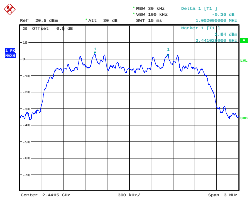
\pi/4 -DQPSK_Middle 1.002MHz
