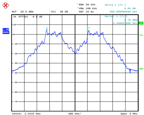
GFSK_Middle 0.999MHz
