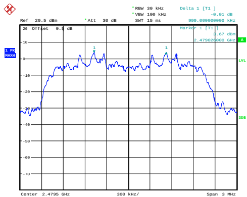
\pi/4 -DQPSK_High 0.999MHz
