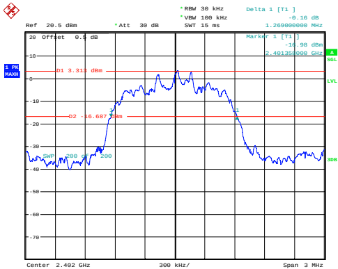
\pi/4 -DQPSK_Low 1.269MHz
