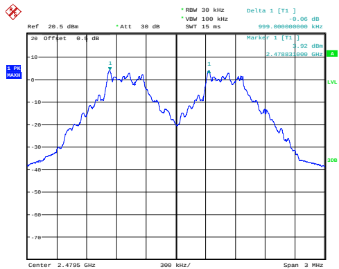
GFSK_High 0.999MHz
