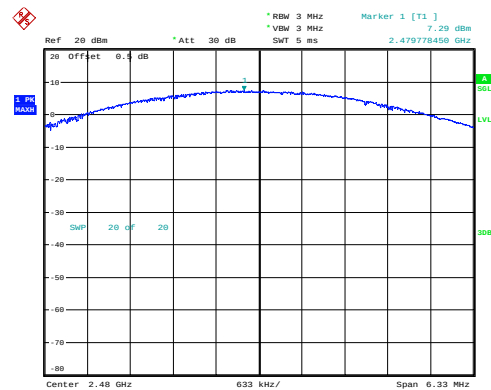
\pi/4 -DQPSK_High 7.29dBm
