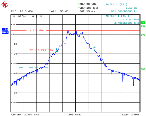
GFSK_Low 0.891MHz
