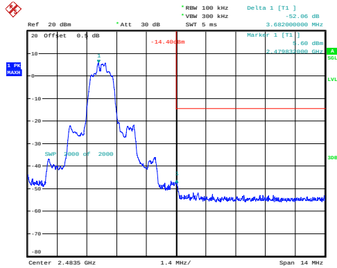
\pi/4 -DQPSK_High 52.06dB
