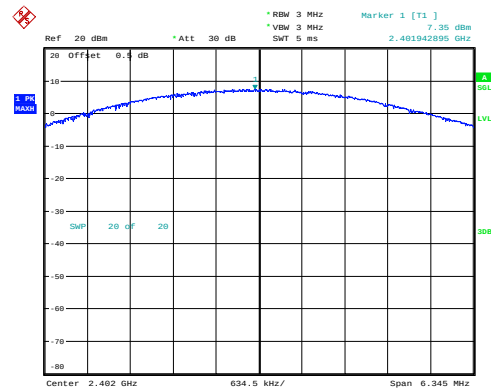
\pi/4 -DQPSK_Low 7.35dBm
