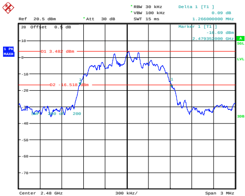
\pi/4 -DQPSK_High 1.266MHz
