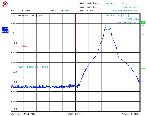
GFSK_Low 57.31dB
